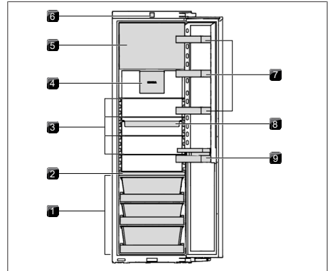
Rys. 5.2 Budowa C178KGF
