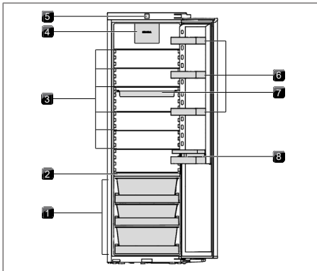
Rys. 5.1 Budowa C178K
