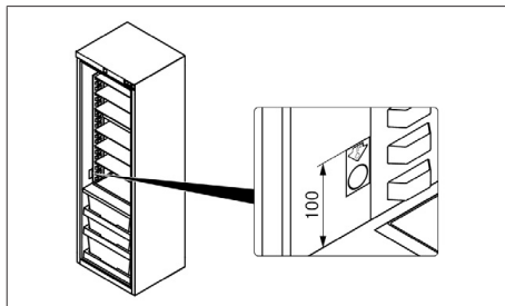
Fig. 8.16 Plassere temperaturindikatoren
