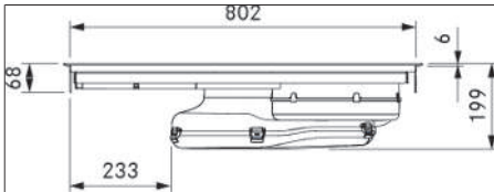
Bild 3.5 PUXU2/R apparatmått bild framifrån
