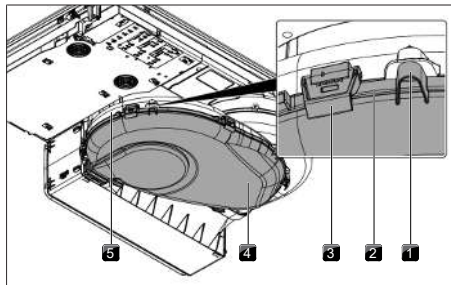
Bild 9.3 Luftledningskåpa
