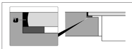
Bild 11.36 Silikontätningssmassa vid planmontering
