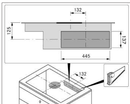
Bild 11.11 Utskärning i den baksidan
