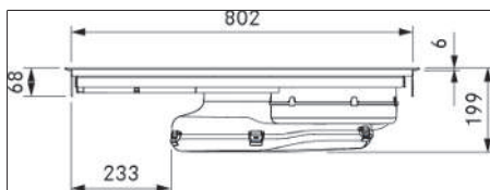
Bild 3.2 PUXA2/R apparatmått bild framifrån
