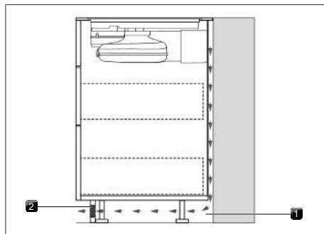
Bild 11.10 Återströmningsöppning i sockelområdet
