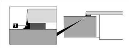
Bild 11.35 Silikontätningssmassa vid ytmontering
