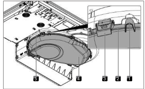
Fig. 9.3 Luftføringsapparatet
