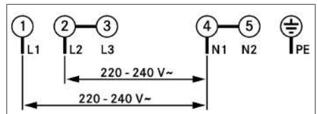
Fig. 11.29 Koblingsskjema 2-fase-tilkobling
