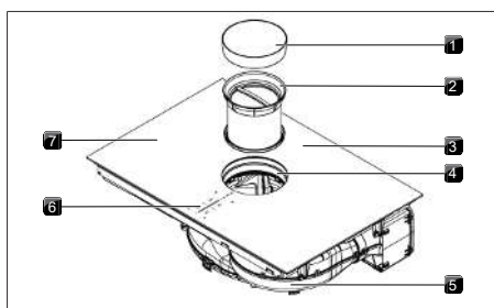
Fig. 4.1 Konstruksjon
