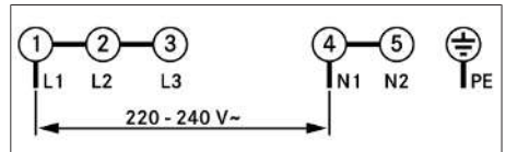
Fig. 11.28 Koblingsskjema 1-fase-tilkobling
