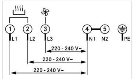
Fig. 11.27 Koblingsskjema 3-fase-tilkobling
