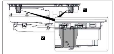
Fig. 11.19 Sette på monteringsklemmer
