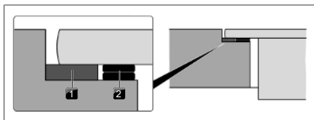
Fig. 11.22 Høydejusteringsplater
