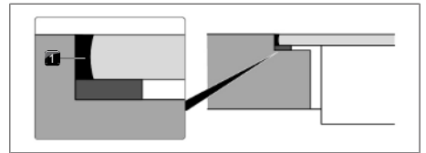
Fig. 11.36 Silikonfugemasse ved planlimt montering
