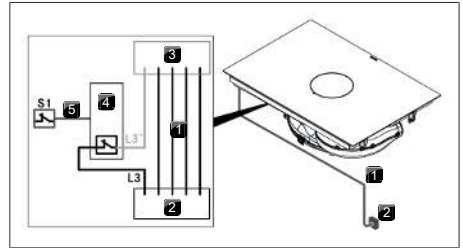
Fig. 11.26 Koblingsskjema med ekstern bryterkontakt
