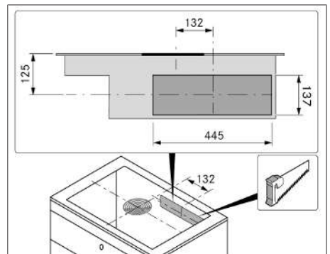
Fig. 11.11 Utskjæring i bakvegg
