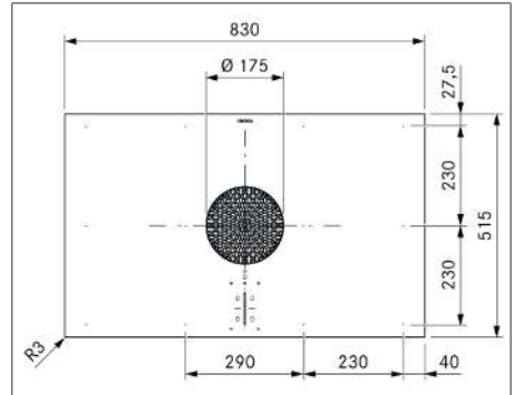
Fig. 3.1 PUXA2/R apparatdimensjoner sett ovenfra
