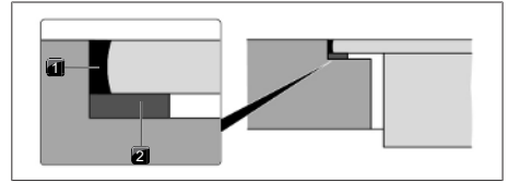
Fig. 11.18 Forseglingsstape ved planlimt montering
