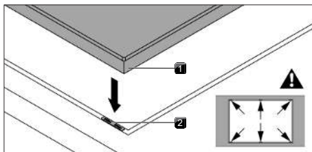
Fig. 11.21 Plassing av høydejusteringsplatene
