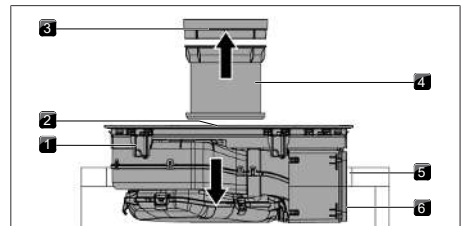
Fig. 11.20 Plasser platetoppen i midten
