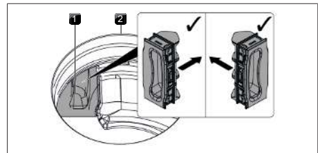
Fig. 9.10 Sette inn klaff for filterskifte
