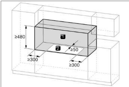
Fig. 11.3 Påkrevd avstand
