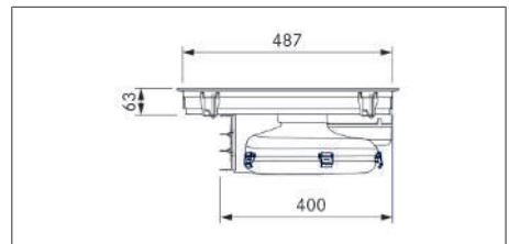
Fig. 3.3 PUXA2/R apparatdimensjoner sett fra siden
