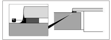
Fig. 11.35 Silikontetningsmasse ved overflatemontering
