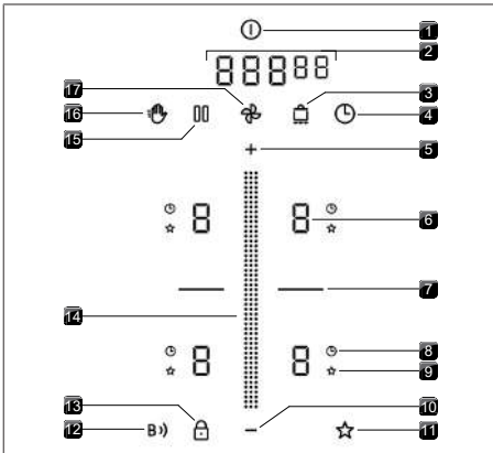
Fig. 4.4 Betjeningsfelt
