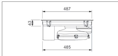
Fig. 3.6 PUXU2/R apparatdimensjoner sett fra siden
