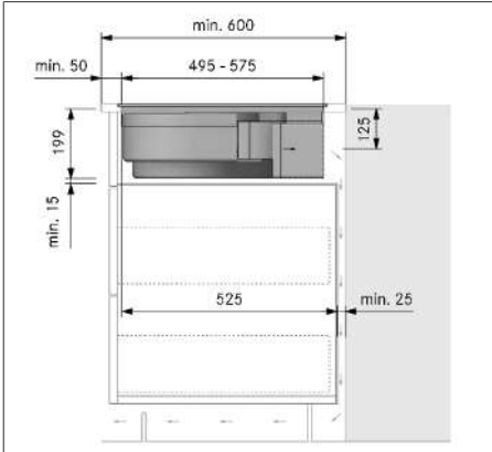
Fig. 11.16 Monteringsdimensjoner ved resirkulering - monteringsvariant B, benkeplatedybde 600 mm
