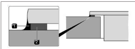
Fig. 11.17 Forseglingsstape ved overflatemontering
