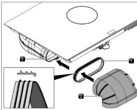
Fig. 11.24 Tilkobling til kanalsystemet
