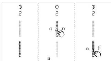
Fig. 8.3 Menypunkt 2: Barnesikring
