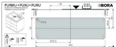
Fig. 11.12 Mål til utskjæring i bakvegg
