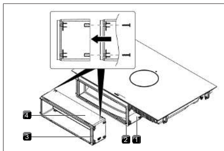
Fig. 11.15 Forlengelse av teleskoputtrekket
