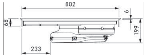
Fig. 3.2 PUXA2/R apparatdimensjoner sett forfra
