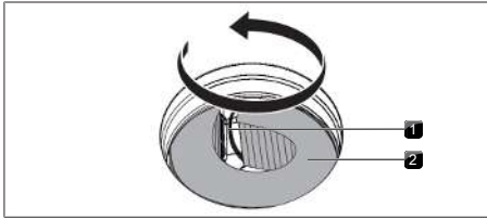
Fig. 9.5 Vri luftfilteret ut av apparathuset
