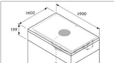
Fig. 11.4 Møbel-minstemål X Pure
