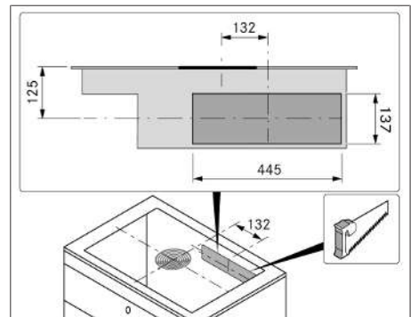
obr. 11.11 Výřez v zadní stěně
