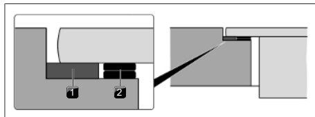
obr. 11.22 Podložky k nastavení výšky
