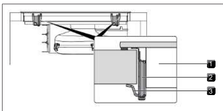
obr. 11.23 Upevnění varné desky do středu
