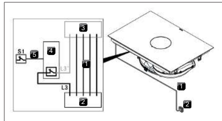
obr. 11.26 Schéma zapojení s externím spínacím kontaktem
