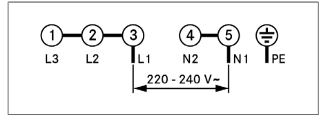
obr. 11.31 Schéma připojení u jednofázové přípojky
