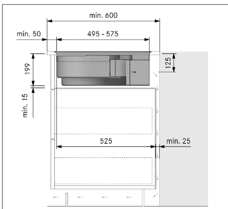
obr. 11.18 Rozměry montáže u varianty montáže B, hloubka pracovní desky 600 mm
