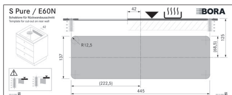
obr. 11.16 Šablona pro výřez zadní stěny
