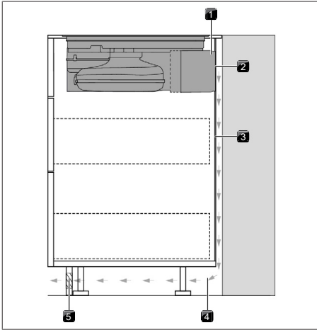
obr. 11.13 Varianta montáže s průchozí zadní stěnou
