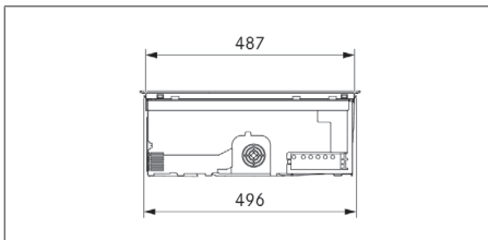
obr. 3.6 Pohled z boku na spotřebič PURSU2/R
