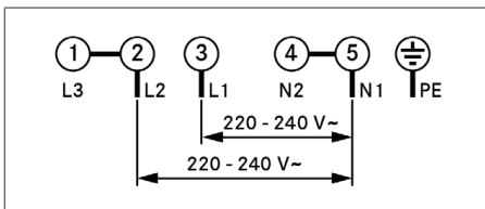
obr. 11.30 Schéma připojení u dvoufázové přípojky
