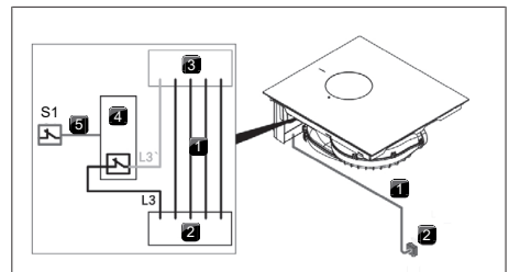
obr. 11.33 Schéma zapojení s externími spínacími kontakty
