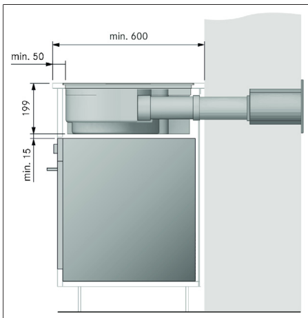
obr. 11.5 PURSA2/R nad troubou s prouděním vzduchu přímo dozadu do pouzdra ve stěně
