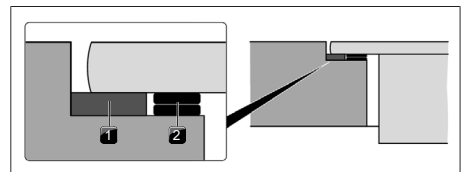
obr. 11.24 Podložky k nastavení výšky
