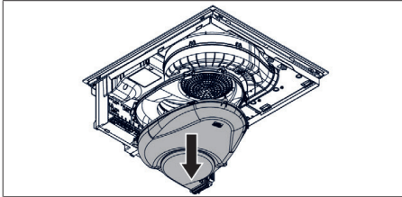
obr. 11.28 Demontáž spodní části sací komory
