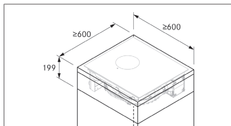
obr. 11.4 Minimální rozměry nábytku – S Pure
