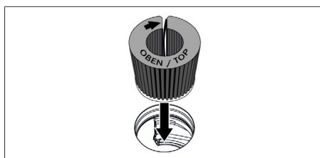
obr. 9.8 Nasazení pachového filtru do otvoru odsavače
