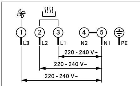
obr. 11.29 Schéma připojení u trojfázové přípojky
