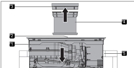
obr. 11.21 Nasazení varné desky
