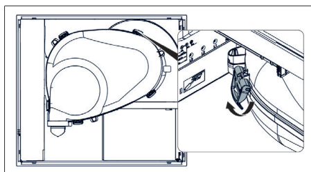
obr. 11.27 Uzávěry sací komory
