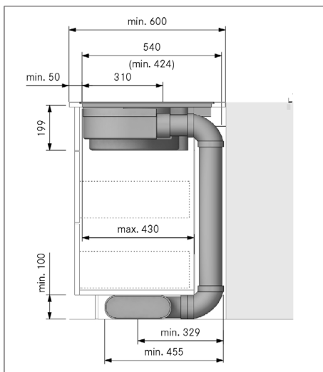
obr. 11.11 Rozměry montáže při odtahu ven, hloubka pracovní desky 600 mm
