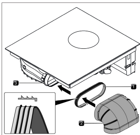
obr. 11.25 Připojení systému odtahových potrubí
