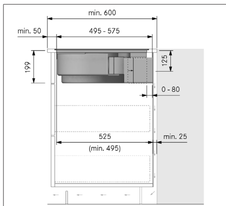
obr. 11.17 Rozměry montáže u recirkulujícího vzduchu, varianta montáže A
