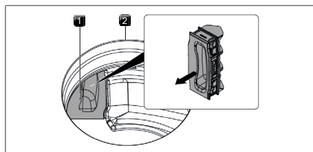
obr. 9.4 Sejmutí výměnné klapky filtru
