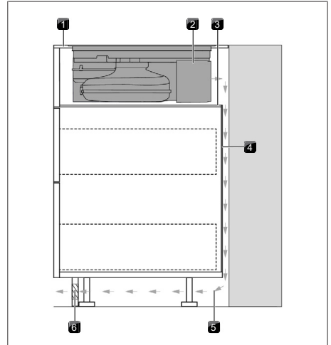
obr. 11.14 Varianta montáže s vloženým dnem
