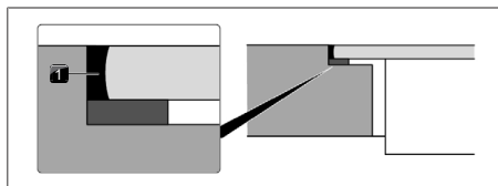
obr. 11.39 Silikonová těsnicí hmota při plošně zarovnané montáži
