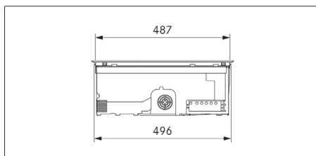
obr. 3.3 Pohled z boku na spotřebič PURSA2/R
