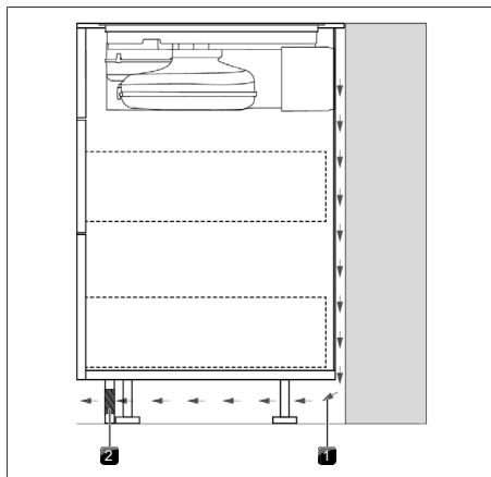
obr. 11.12 Otvor na zpětné proudění vzduchu v oblasti soklu
