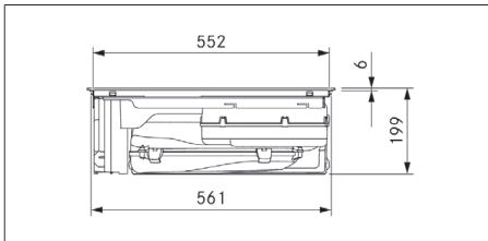
obr. 3.5 Pohled zepředu na spotřebič PURSU2/R
