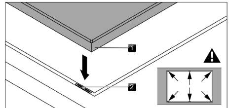
obr. 11.23 Pozice podložek k nastavení výšky
