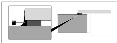
obr. 11.38 Silikonová těsnicí hmota při montáži na povrch
