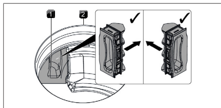
obr. 9.10 Nasazení výměnné klapky filtru
