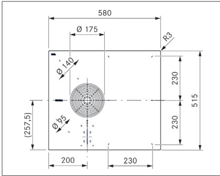
obr. 3.4 Pohled shora na spotřebič PURSU2/R
