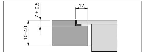
obr. 11.10 Rozměr drážky pro plošně zarovnanou montáž
