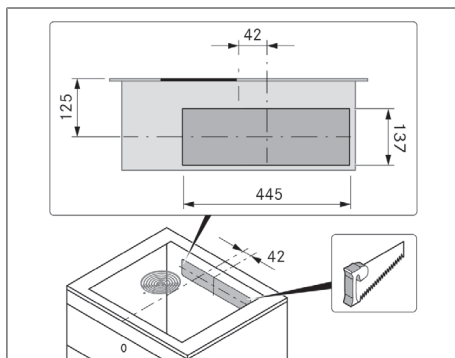
obr. 11.15 Výřez v zadní stěně
