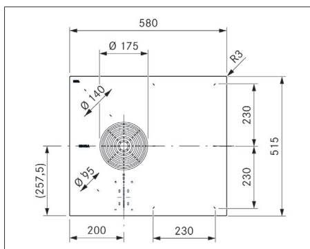
obr. 3.1 Pohled shora na spotřebič PURSA2/R
