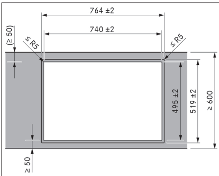
Fig. 11.5 Dimensions de découpe pour montage affleurant
