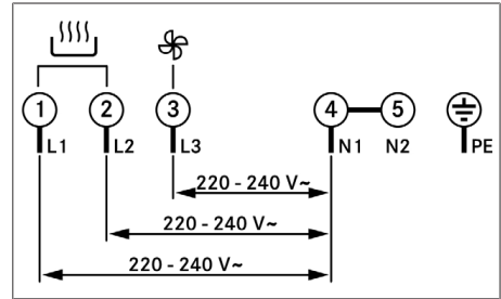
Fig. 11.27 Schéma de raccordement triphasé
