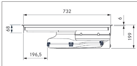
Fig. 3.5 Dimensions PURU2/R - Vue de devant
