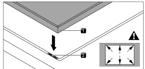
Fig. 11.21 Positionnement des plaques de compensation des hauteurs
