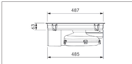
Fig. 3.6 Dimensions PURU2/R - Vue latérale
