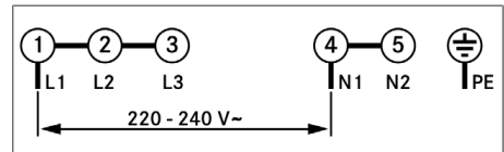
Fig. 11.28 Schéma de raccordement monophasé
