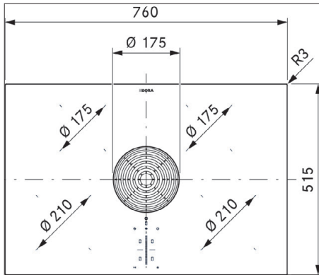
Fig. 3.4 Dimensions PURU2/R - Vue de dessus
