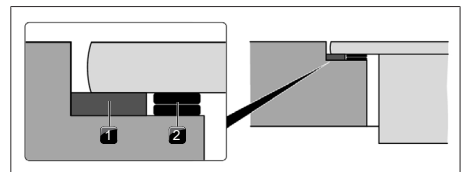
Fig. 11.22 Plaques de compensation des hauteurs
