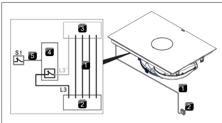
Fig. 11.26 Schéma de raccordement avec contact externe
