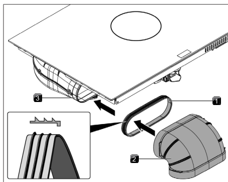
Fig. 11.24 Raccordement au système de canaux
