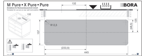
Fig. 11.12 Gabarit de découpe dans la paroi arrière
