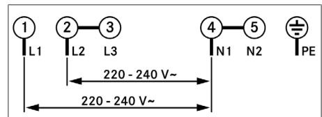
Fig. 11.29 Schéma de raccordement biphasé
