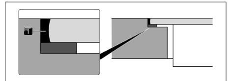
Fig. 11.36 Joint en silicone en montage affleurant
