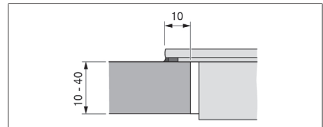
Fig. 11.8 Cote d'appui pour montage en saillie
