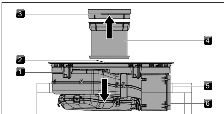
Fig. 11.20 Centrage de la table de cuisson
