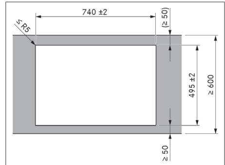
Fig. 11.7 Dimensions de découpe pour montage en saillie
