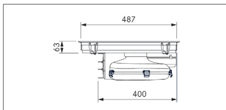
Fig. 3.3 Dimensions PURA2/R - Vue latérale
