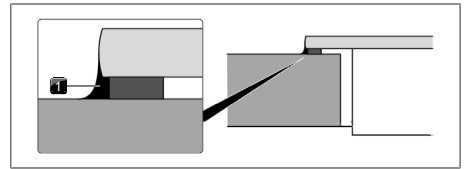
Fig. 11.35 Joint en silicone en montage en saillie
