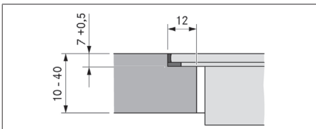
Fig. 11.6 Dimension de rainure pour montage affleurant
