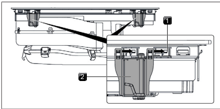
Fig. 11.19 Pose des pinces de montage
