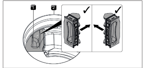
Fig. 9.10 Pose du clapet de changement de filtre
