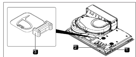
Fig. 11.30 Raccordements électriques de la table de cuisson
