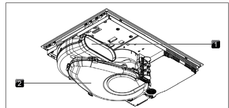
Fig. 4.2 Vue de dessous de la variante à évacuation d'air
