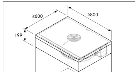
Fig. 11.4 Dimensions minimales du meuble
