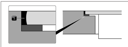
Fig. 11.36 Silikoneforseglingsmassee ved planimet montering
