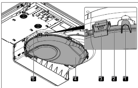
Fig. 9.3 Luftføringskabinettet
