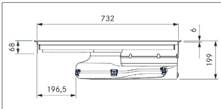
Fig. 3.5 PURU2/R - enhedens mål set forfra
