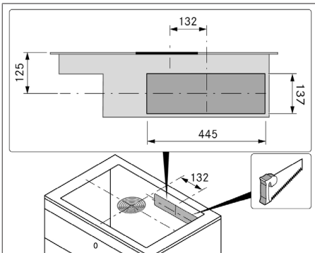
Fig. 11.11 Udsæring i bagvæggen
