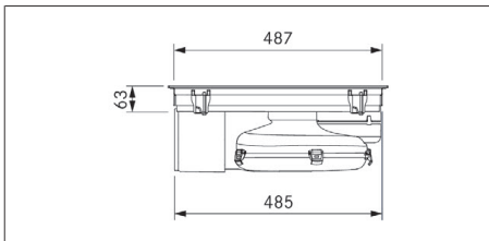
Fig. 3.6 PURU2/R - enhedens mål set fra siden
