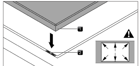
Fig. 11.21 Placering af højdeudligningspladerne
