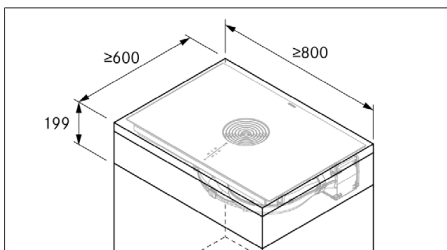
Fig. 11.4 Møbel mindstemål
