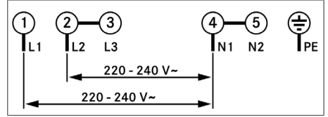
Fig. 11.29 Tilslutningsskema, 2-faset tilslutning
