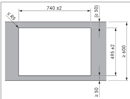
Fig. 11.7 Udskæringsmål til overflademontering
