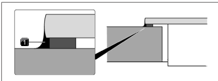
Fig. 11.35 Silikonemassee ved overflademontering
