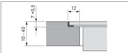
Fig. 11.6 Falsmål til planlimet montering
