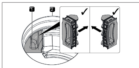
Bild 9.10 Sätta i filterbytesklaffen
