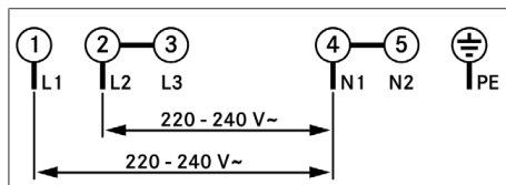
Bild 11.29 Anslutningsschema 2-fas anslutning
