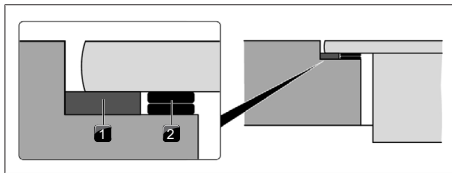
Bild 11.22 Höjdtjämningsplattor
