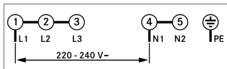
Bild 11.28 Anslutningsschema 1-fas anslutning
