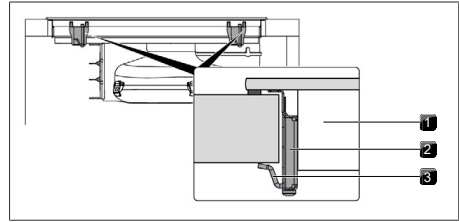
Bild 11.23 Fästa spishällen centrerat
