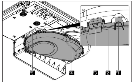
Bild 9.3 Luftledningskåpa
