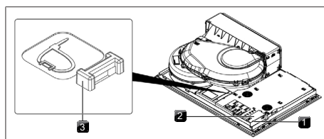
Bild 11.30 Spishällens elektriska anslutningar
