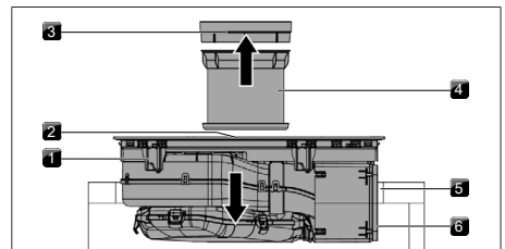
Bild 11.20 Placera spishällen centrerat
