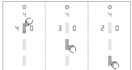
Bild 8.5 Menypunkt 4: Välja tiden för fördröjd avstängning
