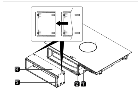
Bild 11.15 Förlängning av teleskoputdraget
