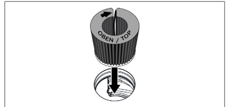
Bild 9.8 Sätta in luftfiltret i ångsugsöppningen
