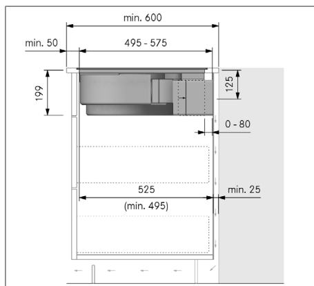
Abb. 11.13 Einbaumaße bei Umluft, Montagevariante A
