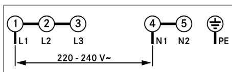
Abb. 11.28 Anschlusschema 1-Phasen-Anschluss
