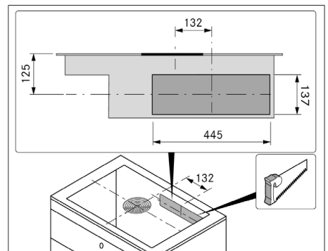
Abb. 11.11 Rückwand-Ausschnitt
