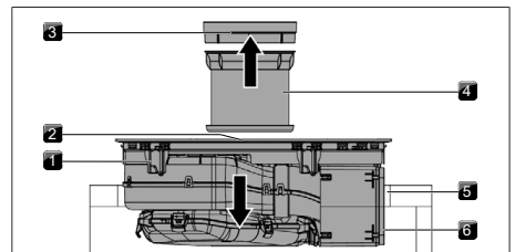
Abb. 11.20 Kochfeld mittig einsetzen
