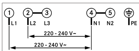
Abb. 11.29 Anschlusschema 2-Phasen-Anschluss
