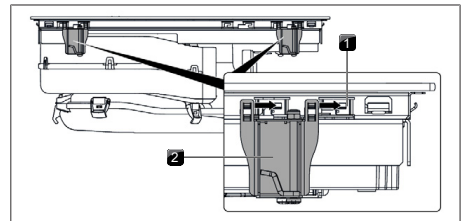
Abb. 11.19 Montageklammern anbringen
