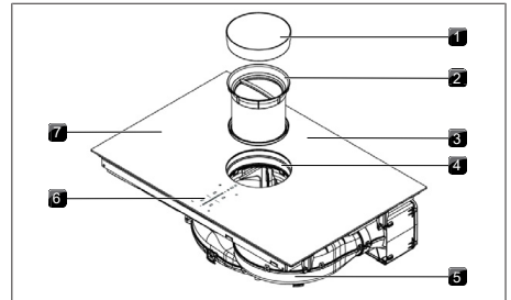
obr. 4.1 Uspořádání
