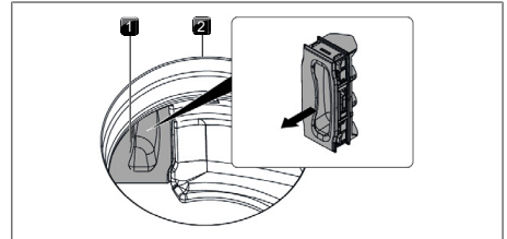
obr. 9.4 Sejmутí výměnné klapky filtru
