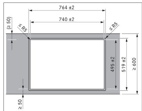
obr. 11.5 Rozměry výřezu pro plošně zarovnanou montáž
