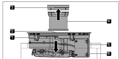
obr. 11.20 Upevnění varné desky do středu
