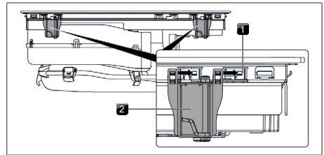
obr. 11.19 Umístění montážních svorek
