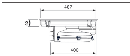
obr. 3.3 Rozměry produktu PURMA2/R – pohled z boku
