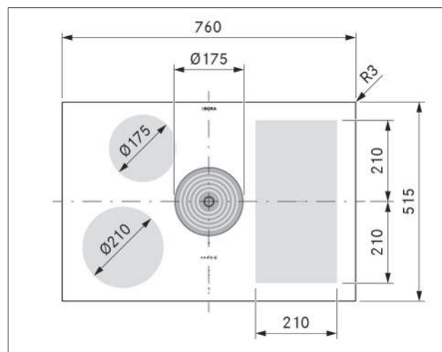
Fig. 3.1 Dimensões do aparelho, vista de cima
