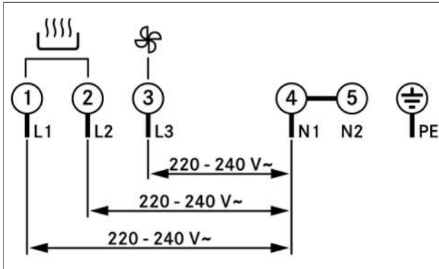
Fig. 9.23 Schéma de raccordement triphasé
