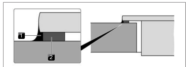
Fig. 9.14 Ruban d'étanchéité pour montage en saillie
