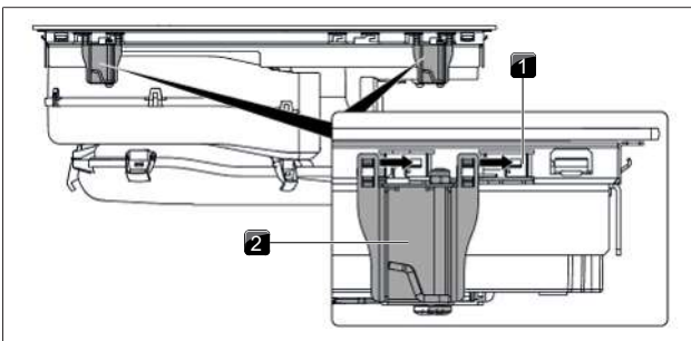
Fig. 9.16 Pose des pinces de montage
