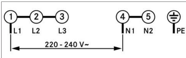
Fig. 9.24 Schéma de raccordement monophasé
