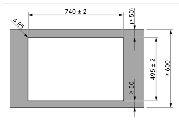
Fig. 9.3 Dimensions de découpe pour montage en saillie
