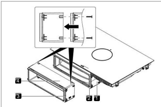
Fig. 9.12 Extension de la section télescopique
