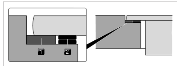
Fig. 9.19 Plaques de compensation des hauteurs
