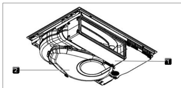
Fig. 4.2 Vue arrière
