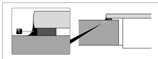
Fig. 9.30 Joint en silicone en montage en saillie
