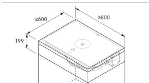
Fig. 9.2 Dimensions minimales du meuble
