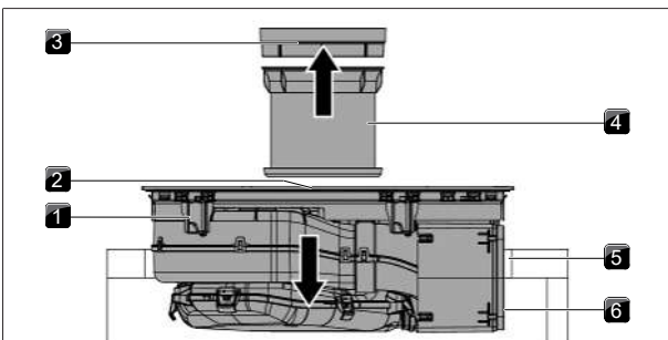
Fig. 9.17 Centrage de la table de cuisson
