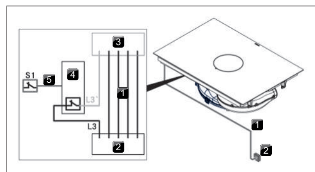
Fig. 9.22 Schéma de raccordement avec contact externe
