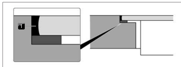
Fig. 9.31 Joint en silicone en montage affleurant
