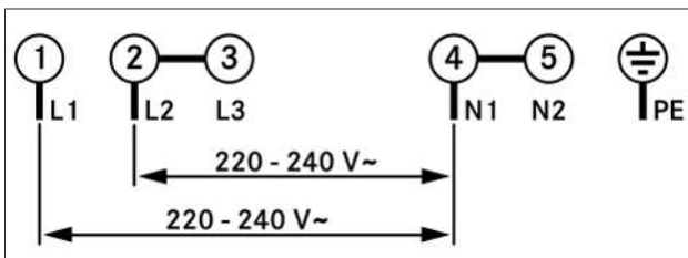
Fig. 9.25 Schéma de raccordement biphasé
