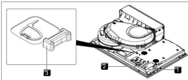
Fig. 9.26 Raccordements électriques de la table de cuisson
