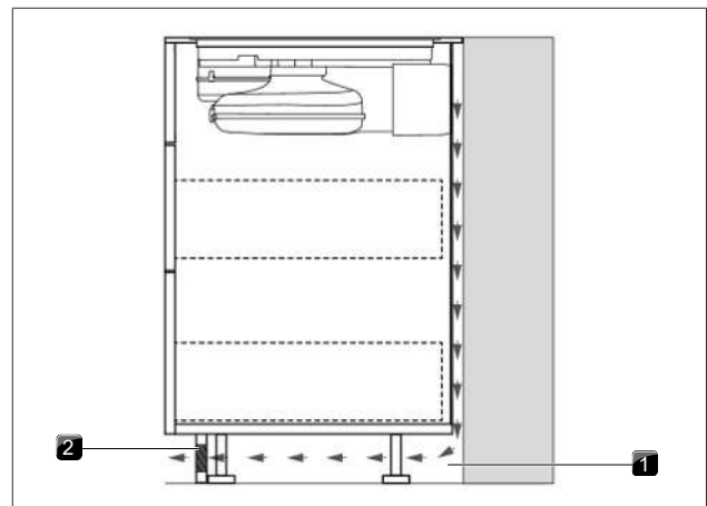
Fig. 9.7 Ouverture de retour de flux dans le socle
