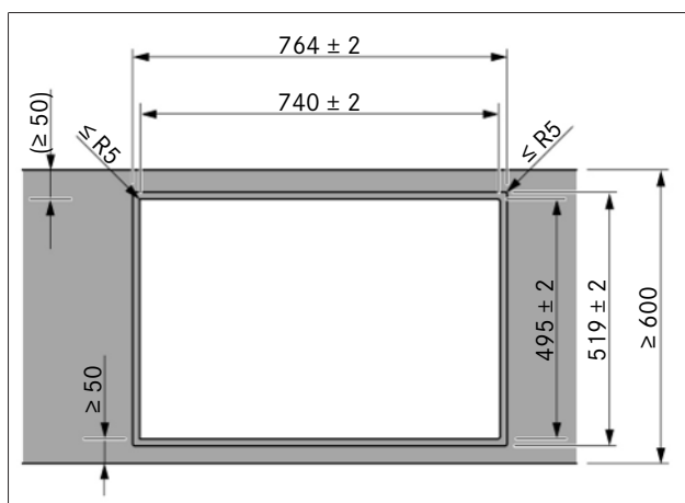
Fig. 9.5 Dimensions de découpe pour montage affleurant
