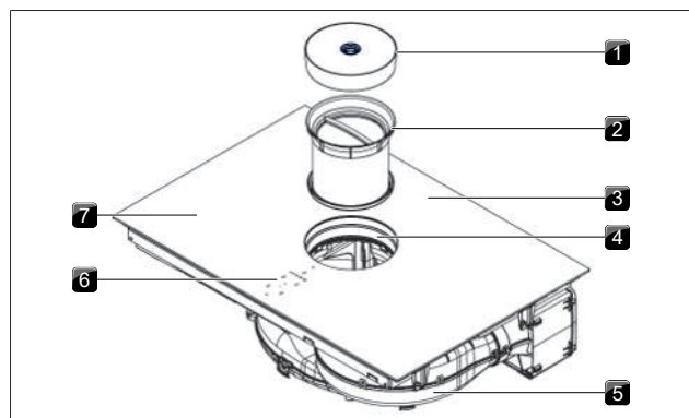
Fig. 4.1 Estructura
