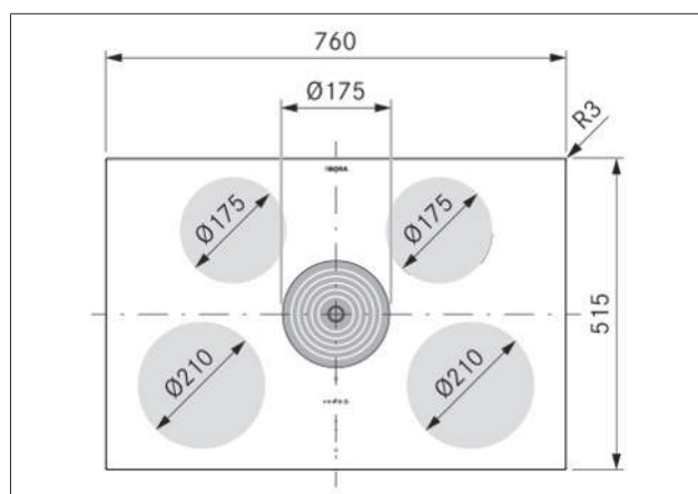
Fig. 3.1 Dimensions de l'appareil - Vue de dessus
