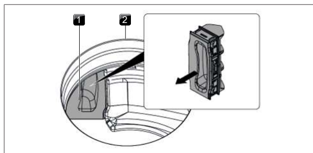
Fig. 7.2 Retrait du clapet de changement de filtre
