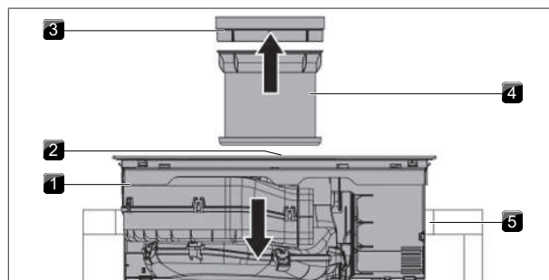
Sl. 9.16 Vstavljanje kuhhalne plošče
