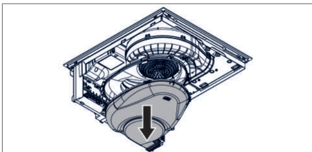
Sl. 9.22 Demontirajte spodnji del sesalne enote.
