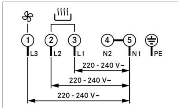
Sl. 9.23 Priključna shema trifaznega priključka
