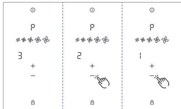
Sl. 9.29 Prikazovalnik točke menija P: Upravljanje moči
