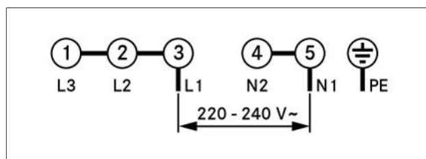
Sl. 9.25 Priključna shema enofaznega priključka
