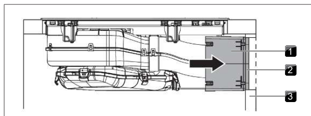
Sl. 9.20 Priključek zadnje strani
