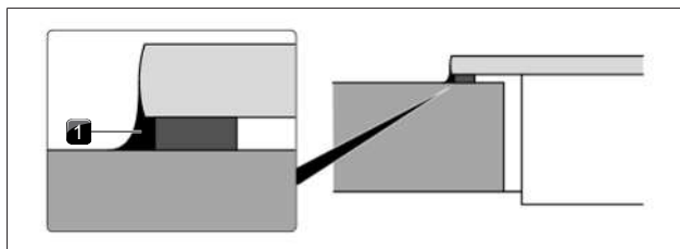
Sl. 9.31 Silikonska tesnilna masa pri nasadni montaži
