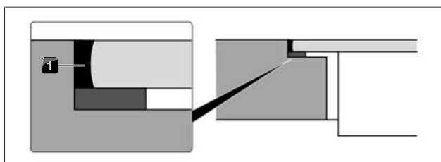
Sl. 9.32 Silikonska tesnilna masa pri montaži v isti ravnini s površino
