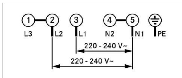
Sl. 9.24 Priključna shema dvofaznega priključka
