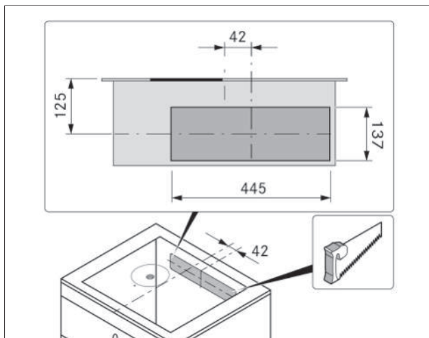
Sl. 9.8 Izrez hrbtišča
