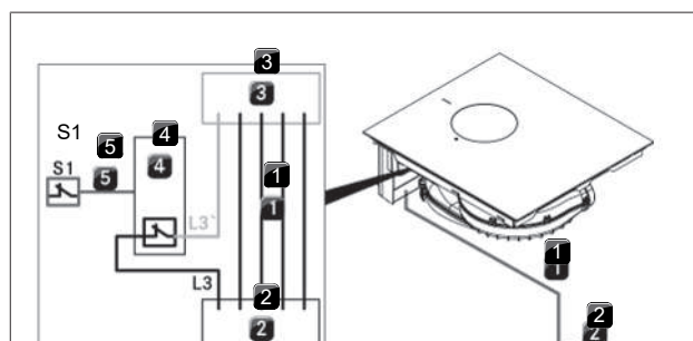
Sl. 9.27 Priključna shema z zunanjiimi stikalnimi kontakti
