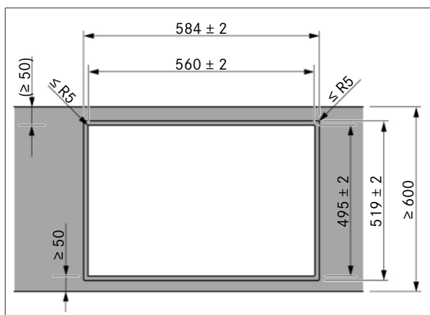
Fig. 9.5 Medidas de recorte para montagem à face
