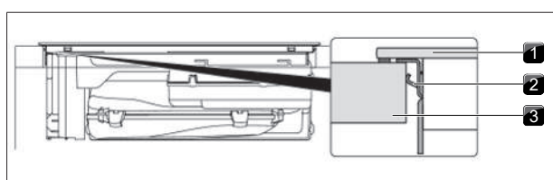
Fig. 9.17 Fixar a placa de cozinhar
