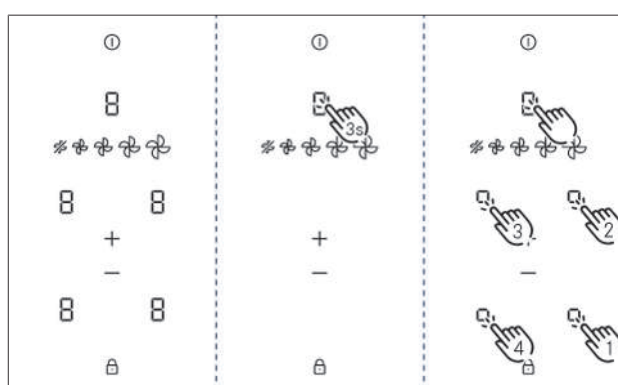
Fig. 9.28 Indicação de como aceder ao menu do distribuidor e de assistência técnica
