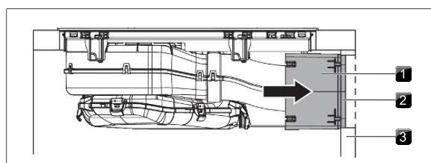
Fig. 9.20 Ligação do painel traseiro
