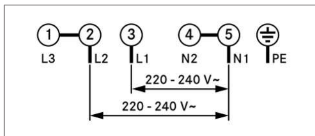
Fig. 9.24 Esquema de ligações para ligação bifásica
