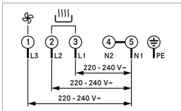
Fig. 9.23 Esquema de ligações para ligação trifásica
