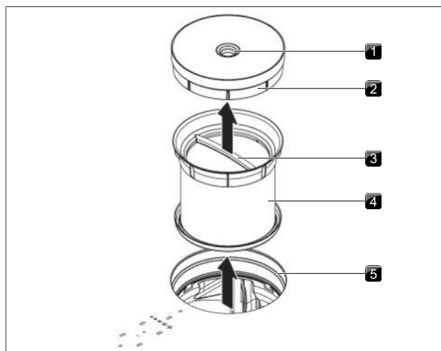
Fig. 7.1 Desmontagem dos componentes
