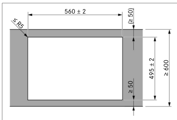
Fig. 9.3 Medidas de recorte para montagem por sobreposição
