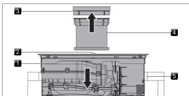
Fig. 9.16 Colocar a placa de cozinhar
