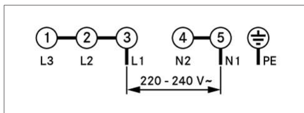
Fig. 9.25 Esquema de ligações para ligação monofásica
