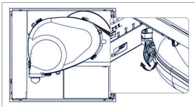
Fig. 9.21 Fechos da câmara de aspiração
