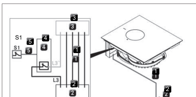
Fig. 9.27 Esquema de ligação com comutadores externos
