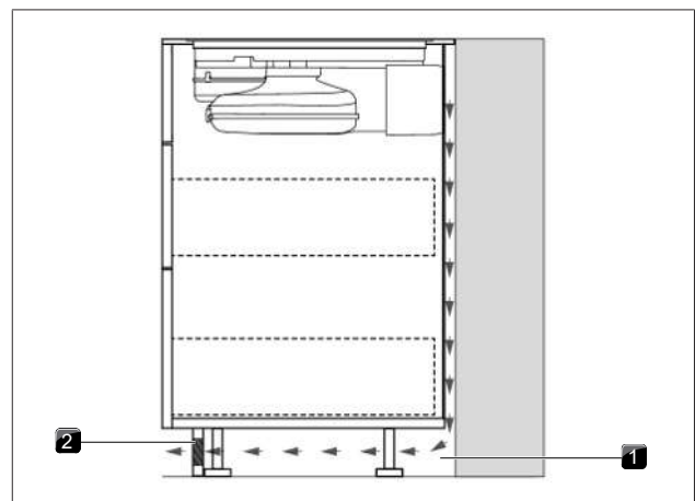
Fig. 9.7 Abertura de retorno na zona de rodapé
