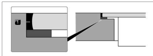
Fig. 9.32 Massa vedante de silicone na montagem à face
