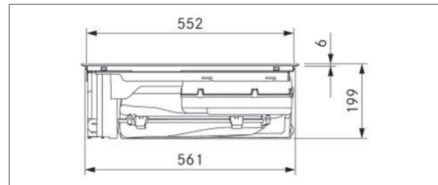
Fig. 3.2 Dimensões do aparelho, vista frontal
