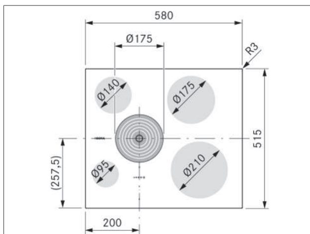
Fig. 3.1 Dimensões do aparelho, vista de cima
