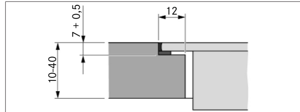
Fig. 9.6 Medida de recesso para montagem à face
