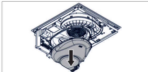
Fig. 9.22 Desmontar a parte inferior da câmara de aspiração.
