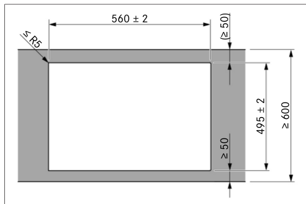
Fig. 9.3 Utskjæringsmål for overflatemontering
