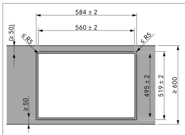
Fig. 9.5 Utskjæringsmål for planlimt montering
