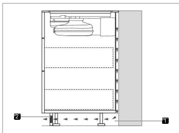
Fig. 9.7 Tilbakestrømningsåpning i sokkelområdet
