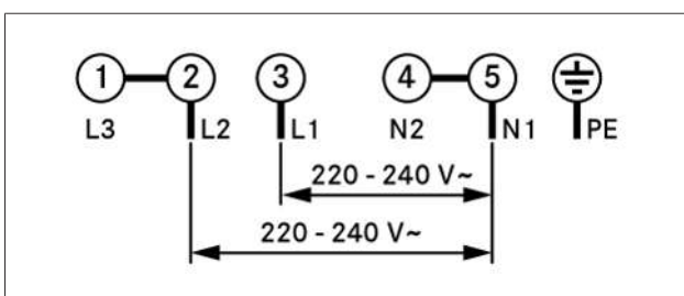
Fig. 9.24 Koblingsskjema tofasekobling
