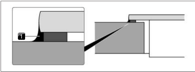
Fig. 9.31 Silikontetningsmasse ved overflatemontering
