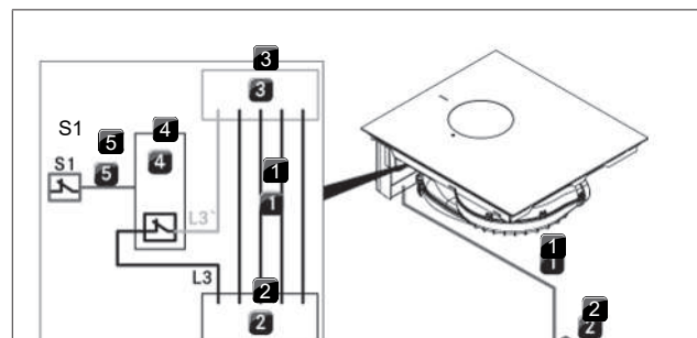
Fig. 9.27 Koblingsskjema med eksterne bryterkontakter
