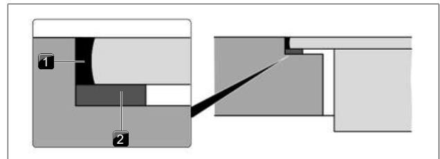
Fig. 9.15 Forseglingstape ved planlimt montering
