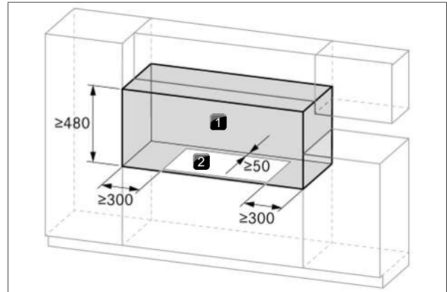
Fig. 9.1 Påkrevd avstand
