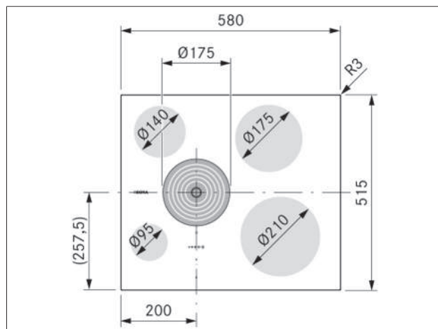
Fig. 3.1 Apparatdimensjoner sett ovenfra
