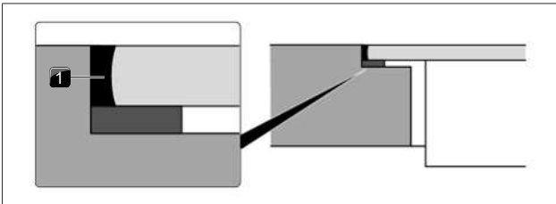
Fig. 9.32 Silikonfugemasse ved planlimt montering
