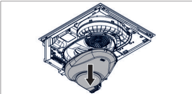
Fig. 9.22 Demonter underdelen av innsugsrommet
