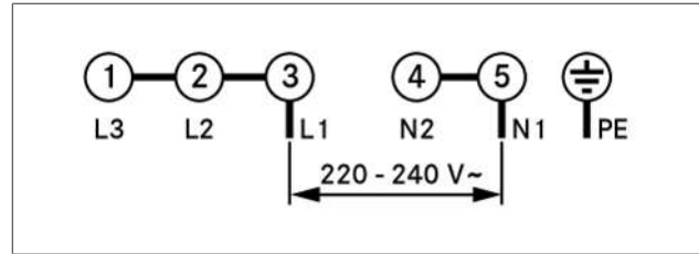
Fig. 9.25 Koblingsskjema enfasekobling
