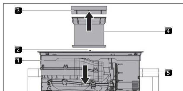
Fig. 9.16 Sette inn platetoppen
