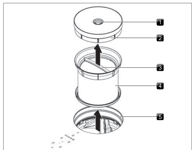
Fig. 7.1 Demontere komponentene
