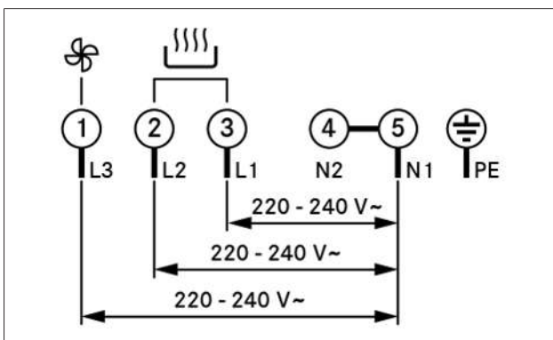
Fig. 9.23 Koblingsskjema trefasekobling
