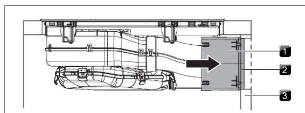
Fig. 9.20 Connessione parete posteriore
