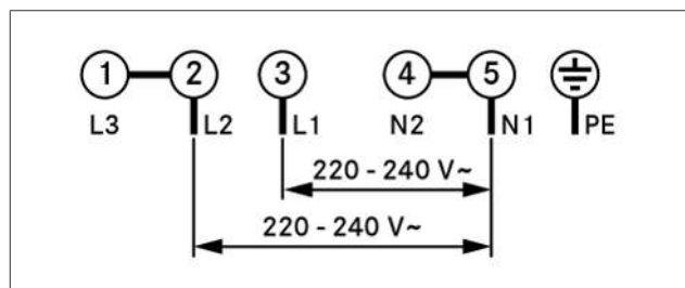
Fig. 9.24 Schema di collegamento connessione bifase
