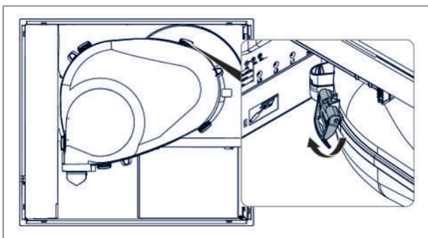
Fig. 9.21 Chiusure del sistema di aspirazione
