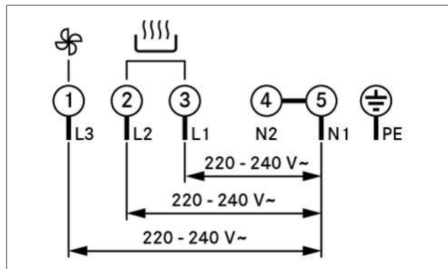
Fig. 9.23 Schema di collegamento connessione a trifase
