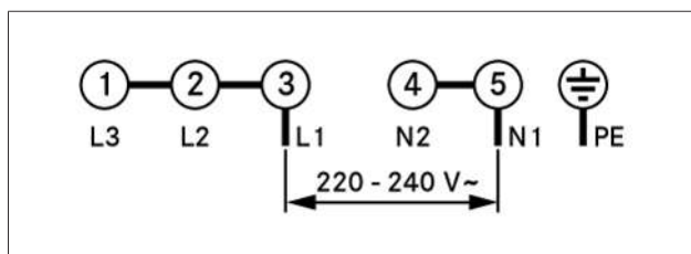
Fig. 9.25 Schema di collegamento connessione monofase
