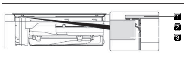
Fig. 9.17 Fissare il piano cottura
