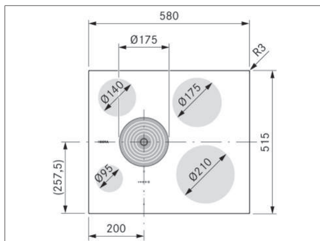
Fig. 3.1 Dimensioni apparecchio vista dall'alto
