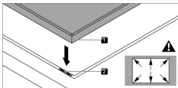
Fig. 9.18 Applicare i pannelli di compensazione altezza
