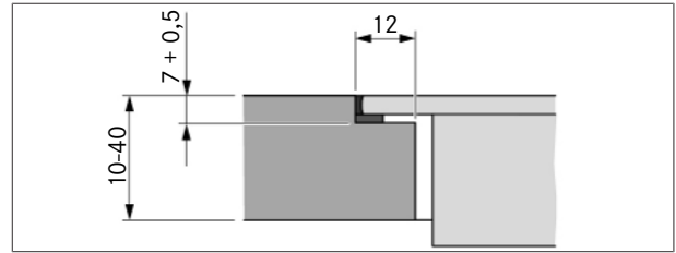
Fig. 9.6 Dimensioni dell'incassatura per montaggio a filo piano
