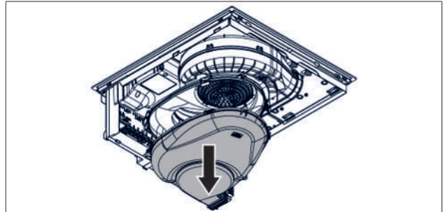
Fig. 9.22 Smontare la parte inferiore del sistema di aspirazione
