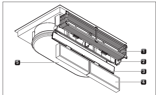
Abb. 5.2 Kochfeldabzug Umluft (BFU)
