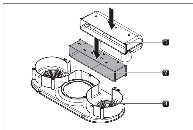
Abb. 6.29 Abluftkanalverlängerung einsetzen
