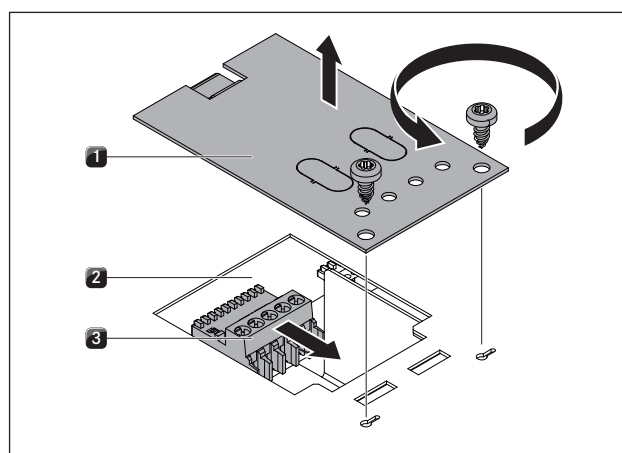
Abb. 6.41 Deckel öffnen und Kontaktstecker abziehen
