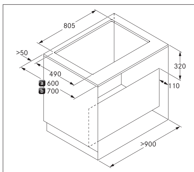
Abb. 6.21 Möbelmaße bei Abluft
