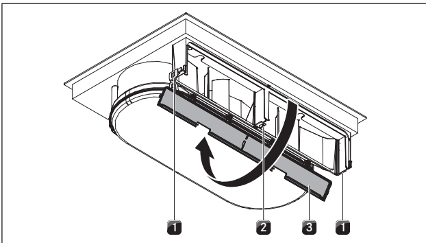
Abb. 6.14 Gehäusedeckel öffnen
