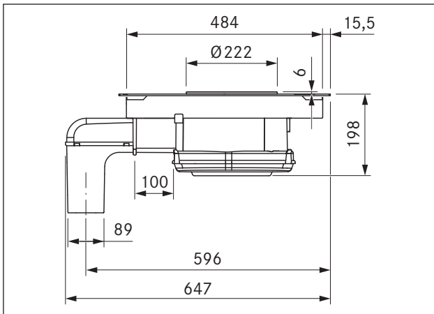
Abb. 3.4 BFI A Gerätemaße Seitenansicht mit horizontaler Abluftkanalverlängerung BLAVH1
