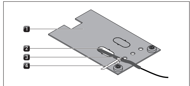
Abb. 6.44 Zugentlastung anbringen
