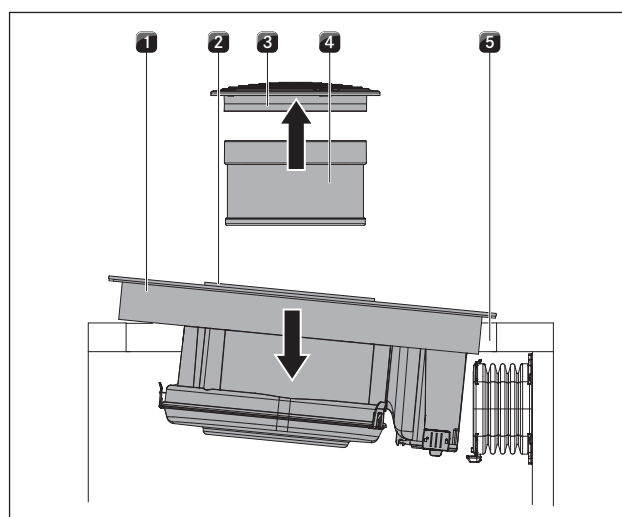
Abb. 6.13 Kochfeld schräg einsetzen
