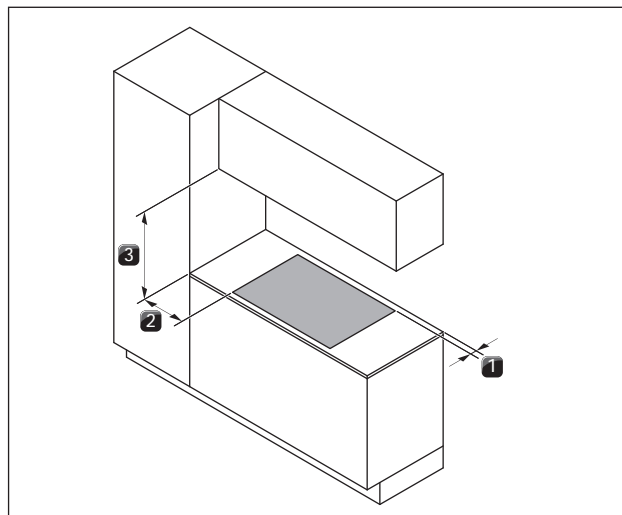
Abb. 6.1 Empfohlene Mindestabstände
