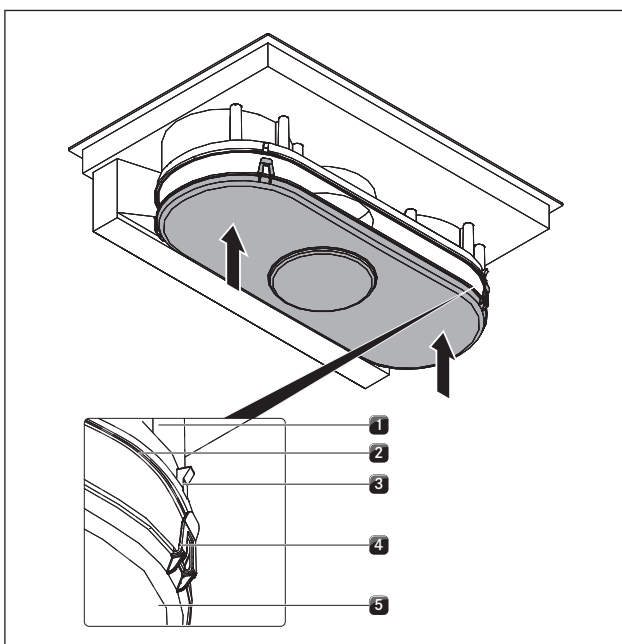
Abb. 8.4 Luftführungsgehäuse schließen
