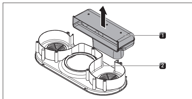
Abb. 6.28 Abluftbogen abnehmen
