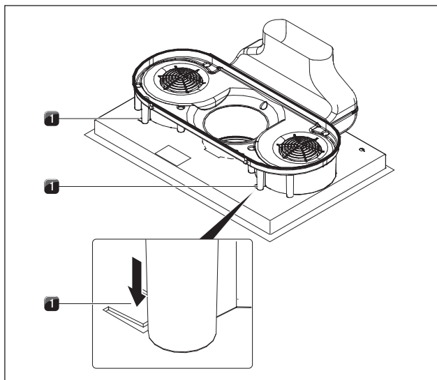
Abb. 6.25 Lagesicherung entriegeln
