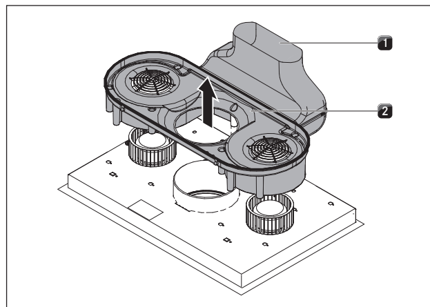
Abb. 6.27 Luftführungsgehäuse abnehmen
