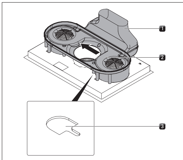
Abb. 6.26 Luftführungsgehäuse verschieben
