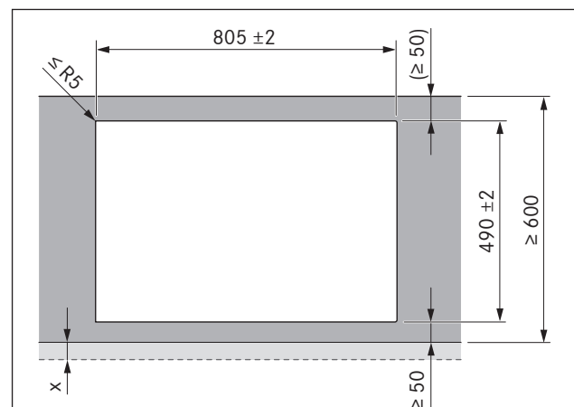
Abb. 6.5 Ausschnittsmaße für Aufsatzmontage
