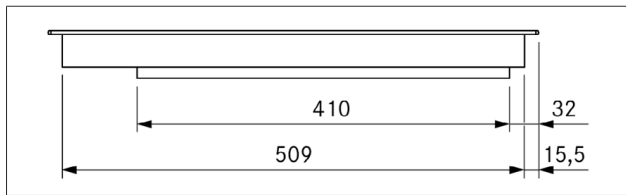
Obr. 3.10 Rozmery spotrebiča PKFI3/PKFI3R, pohľad z boku
