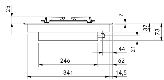
Obr. 3.30 Rozmery varnej dosky PKG3, pohľad spredu
