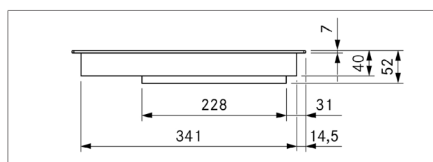
Obr. 3.9 Rozmery spotrebiča PKFI3/PKFI3R, pohľad spredu
