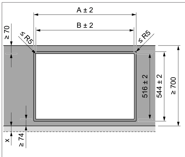
Obr. 4.11 Rozmery výrezu pre zapustenú montáž
