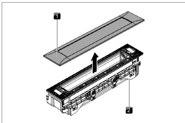
Obr. 4.30 Demontáž krycieho rámu
