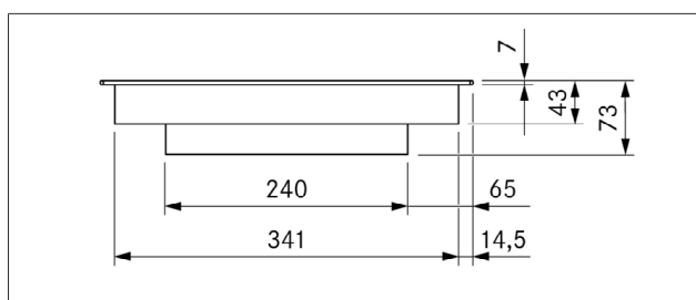
Obr. 3.24 Rozmery varnej dosky PKCH3, pohľad spredu
