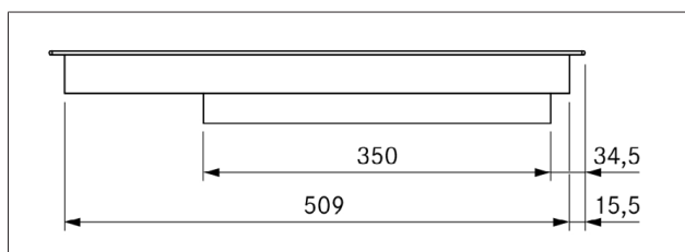
Obr. 3.25 Rozmery varnej dosky PKCH3, pohľad z boku
