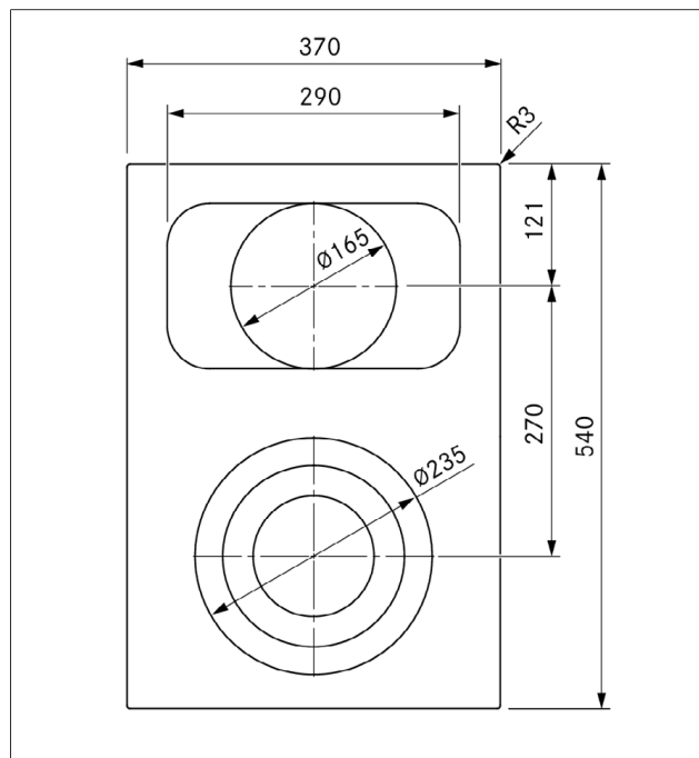
Obr. 3.20 Rozmery varnej dosky PKCB3, pohľad zhora
