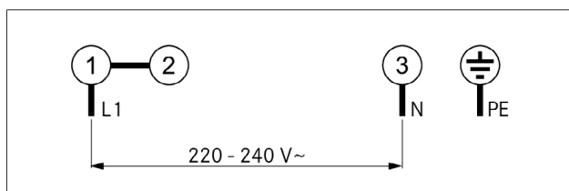
Obr. 4.85 Schéma zapojenia 1-fázová
