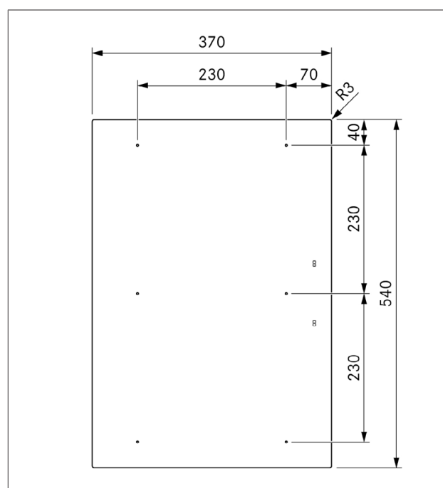
Obr. 3.8 Rozmery spotrebiča PKFI3/PKFI3R, pohľad zhora
