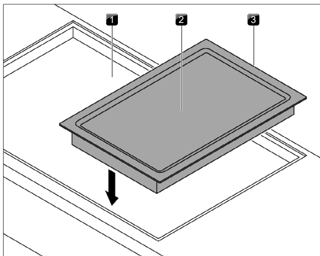
Obr. 4.53 Vloženie Tepan grilu z nerezovej ocele
