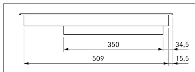
Obr. 3.19 Rozmery varnej dosky PKC3, pohľad z boku
