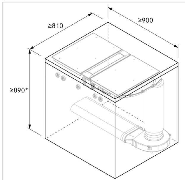
Obr. 4.4 Minimálne montážne rozmery pri štandardnej konštrukcii
