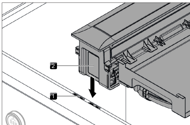
Obr. 4.32 Podložky pre nastavenie výšky
