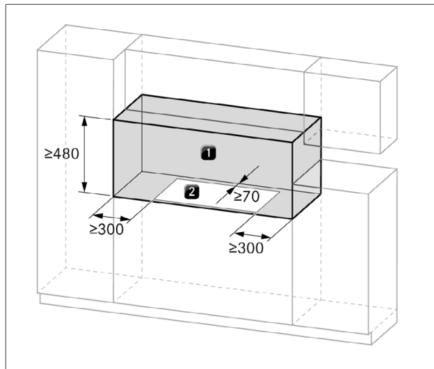
Obr. 4.55 Potrebný voľný priestor
