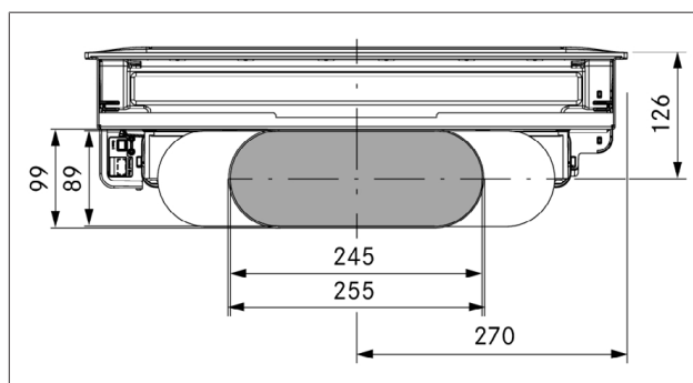
Obr. 4.39 Rozmery pripojenia potrubia PKA3/PKA3AB s kolenovou potrubnou priediodkou
