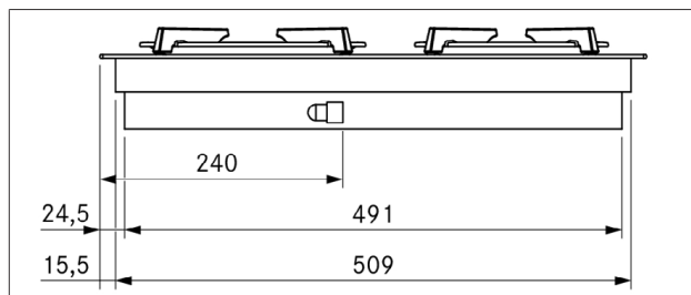
Obr. 3.31 Rozmery varnej dosky PKG3, pohľad z boku
