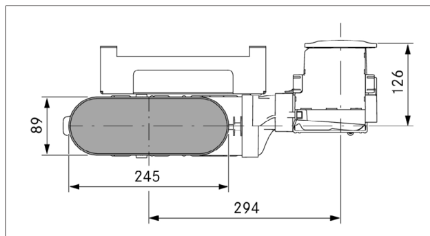
Obr. 4.38 Rozmery pripojenia potrubia PKA3/PKA3AB s kolenovou potrubnou priediodkou
