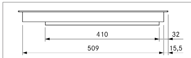
Obr. 3.13 Rozmery varnej dosky PKI3, pohľad z boku
