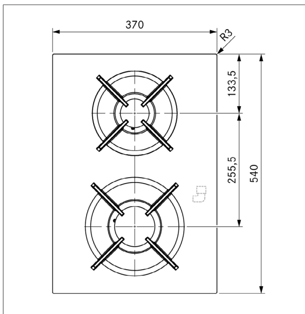
Obr. 3.29 Rozmery varnej dosky PKG3, pohľad zhora
