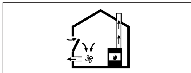
Obr. 4.2 Montáž odvodu vzduchu – správna
