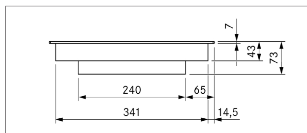
Obr. 3.18 Rozmery varnej dosky PKC3, pohľad spredu
