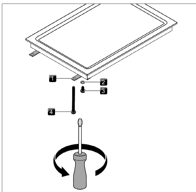
Obr. 4.54 Upevňovacie svorky
