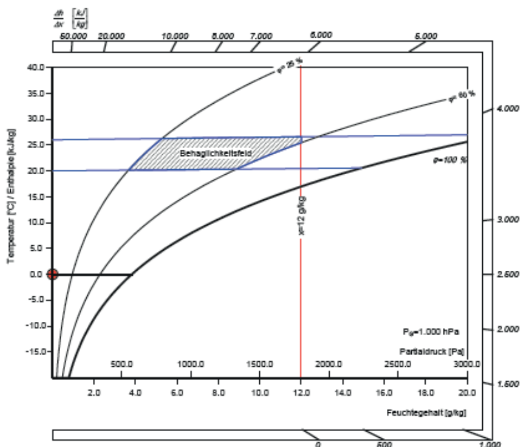
Abb. 3.3-1 Behaglichkeitsbereich nach DIN EN 15 251, Kategorie II [3-6]
