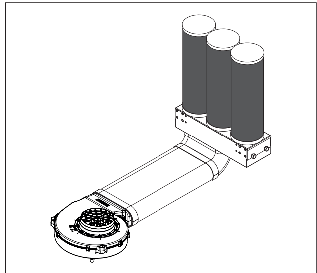
Afb. 4.1 Luchtreinigingsbox in ingebouwde toestand
