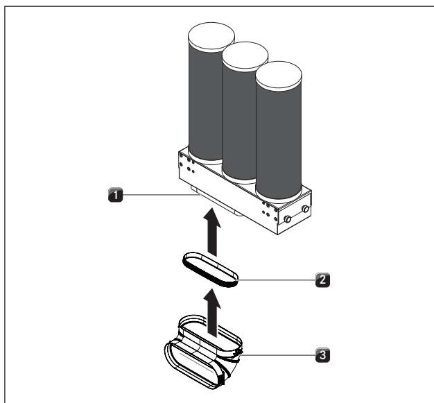
Afb. 4.2 Aansluiting BORA Ecotube kanaalsysteem
