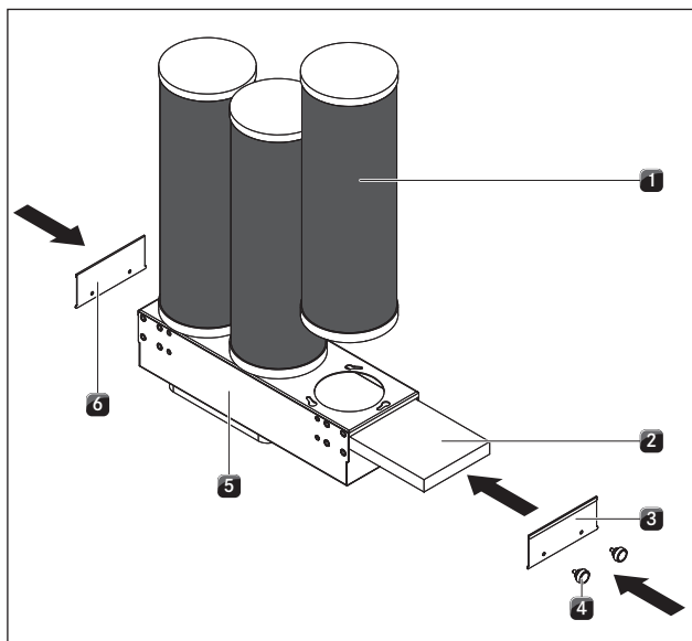
Afb. 3.1 BORA luchtreinigingsbox met 3 actieve-koolfilters (ULB3)
