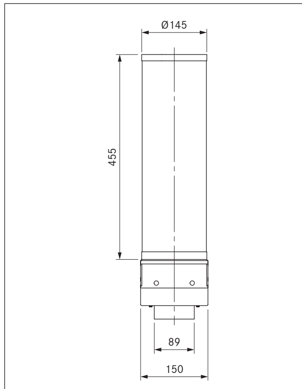
Afb. 3.3 ULB3 Zijaanzicht
