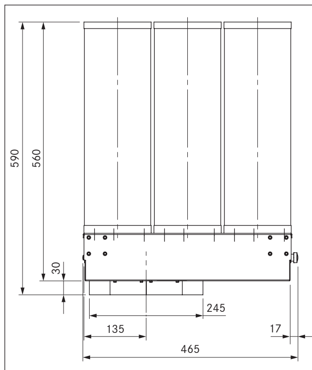
Obr. 3.2 Pohled zepředu ULB3
