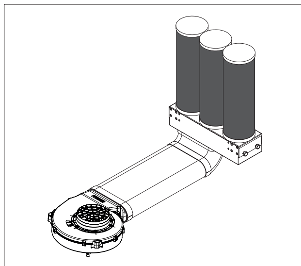
Obr. 4.1 Jednotka čističky vzduchu v zabudovaném stavu
