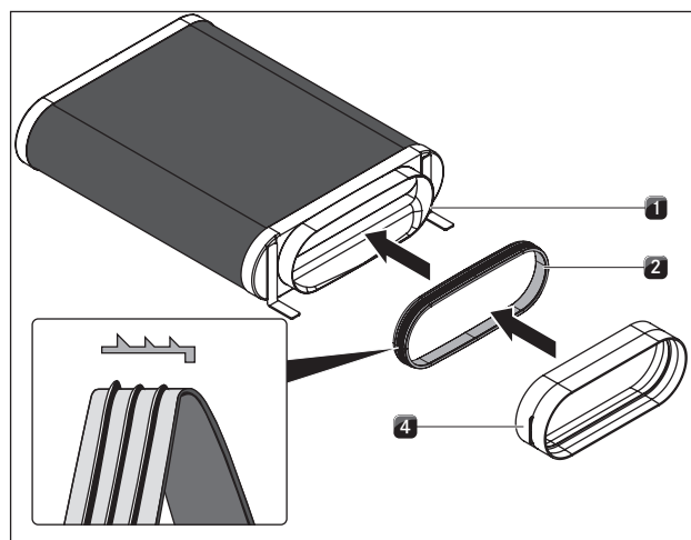
Sl. 4.1 Priključek sistema kanala BORA Ecotube (povezovalec kanala Ecotube ali del modela Ecotube)
