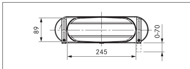
Sl. 3.2 ULB1 pogled od zgoraj
