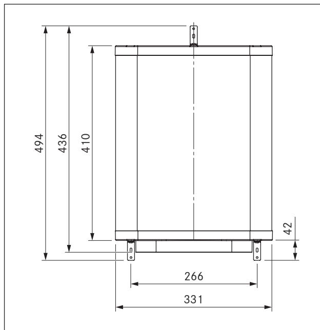
Sl. 3.3 ULB1 pogled od spredaj
