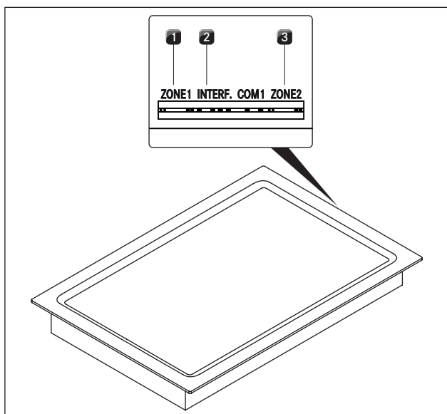
рис. 5.18 Соединение для поворотной ручки управления на задней стороне варочной панели
