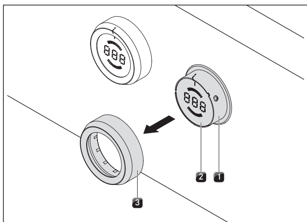
рис. 7.5 Снятие кольца поворотной ручки управления
