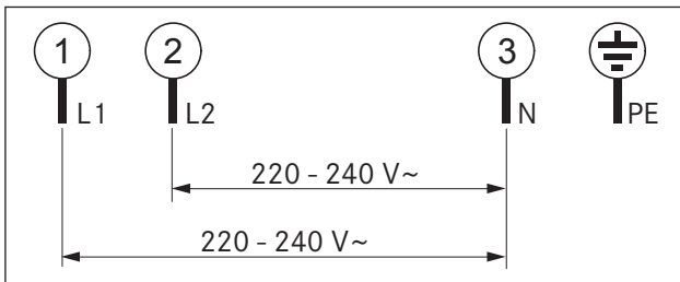
Kuva 5.21 Liitäntäkaavio - 2-vaiheinen liitäntä
