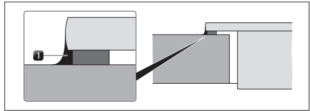
Kuva 5.16 Silikonitiivistysmassa pinta-asennuksessa
