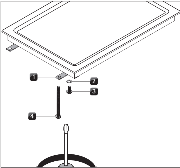
Kuva 5.14 Asennuskannakkeet
