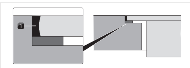
Kuva 5.15 Silikonitiivistysmassa uppoasennuksessa
