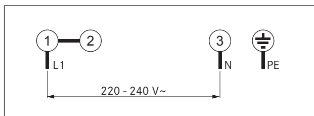
Fig. 5.22 Tilslutningsskema, 1-faset
