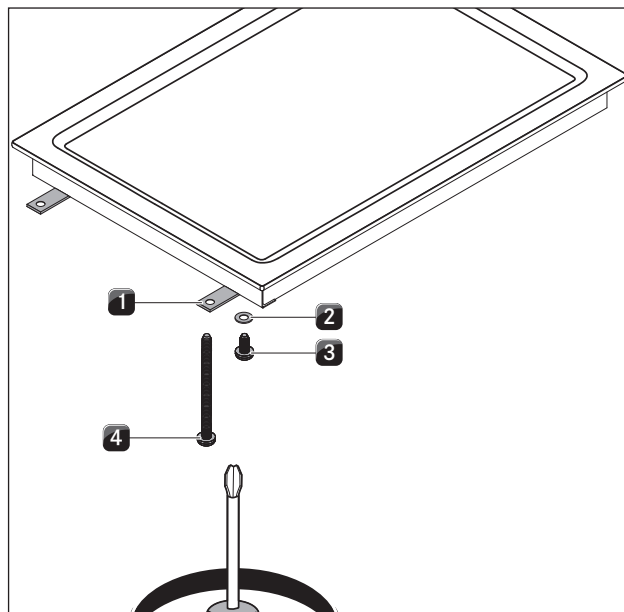
bild 5.16 Fästklammer
