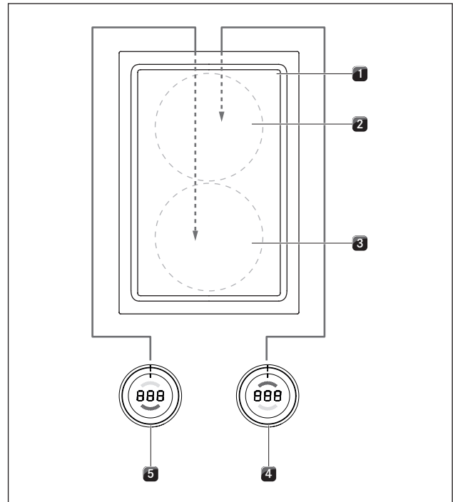
bild 5.19 Kokzonernas standardanslutning
