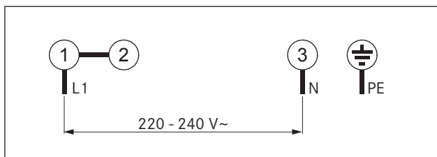
bild 5.23 Anslutningsschema 1-fasigt
