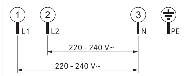
bild 5.22 Anslutningsschema 2-fasigt
