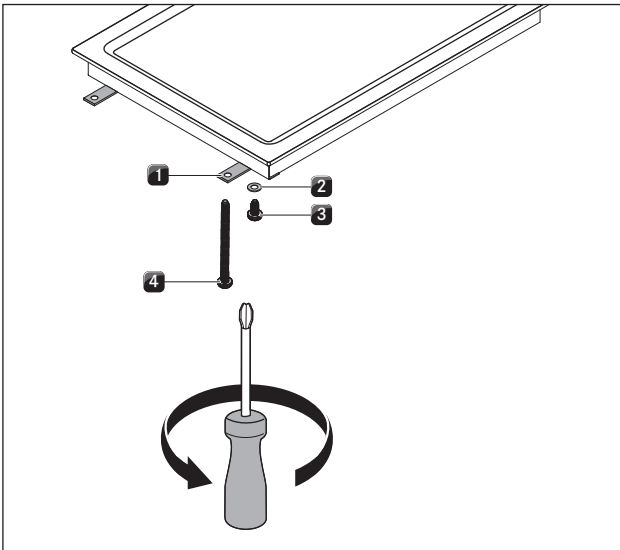
Afb. 5.18 Bevestigingsklemmen
