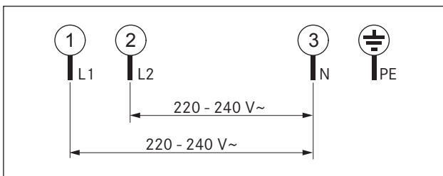
Afb. 5.25 Aansluitschema 2-fasig
