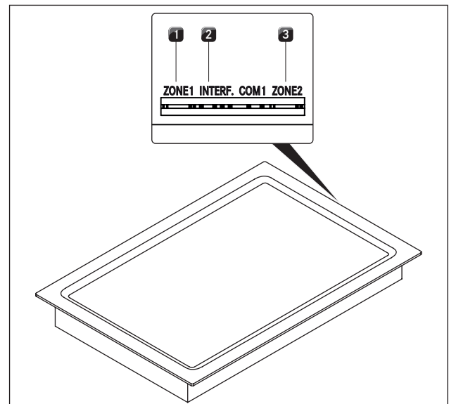
Afb. 5.20 Aansluiting bedieningsknop aan de achterzijde van het kookveld
