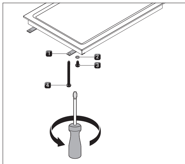
bild 5.18 Fästklämmor
