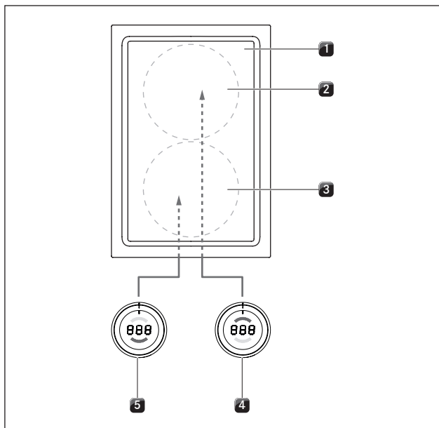
bild 5.22 Anslutning av kokzonerna vid 180° inbyggnad och där apparaterna har anslutningen bak (PKT3)
