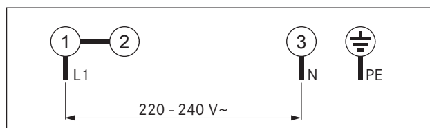
bild 5.24 Kopplingsschema 1-fasigt
