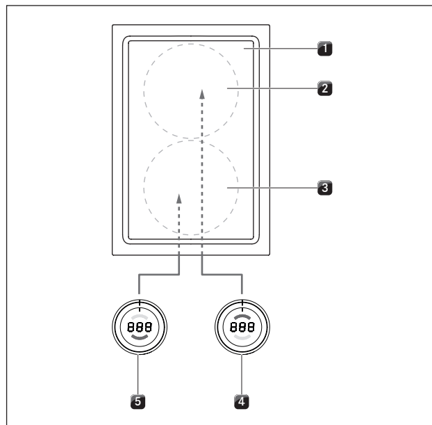
Fig. 5.22 Collegamento delle zone cottura con montaggio girato di 180° e apparecchi con connessione posteriore (PKT3)
