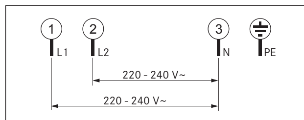
Fig. 5.25 Schema di collegamento bifase
