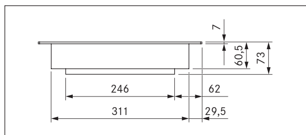
Fig. 3.2 PKT3 dimensioni apparecchio vista frontale
