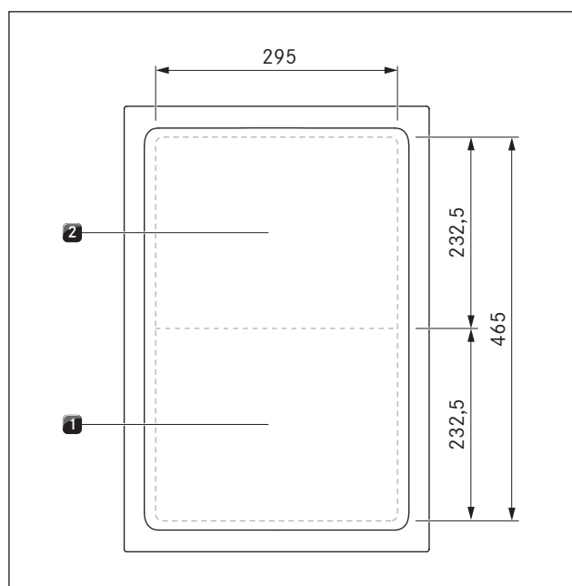
Fig. 4.5 Montaggio griglia Teppanyaki in acciaio inox PKT3 e dimensioni delle zone cottura
