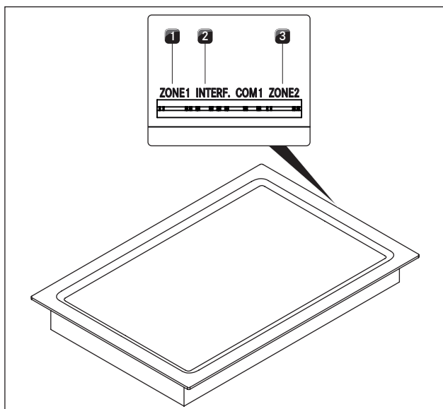
Fig. 5.20 Collegamento manopola di comando sul lato posteriore del piano cottura
