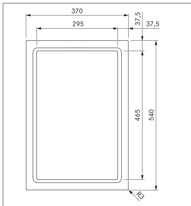
Fig. 3.1 PKT3 dimensioni apparecchio vista dall'alto
