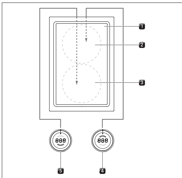
Fig. 5.21 Collegamento standard degli apparecchi con connessione posteriore (PKT3)
