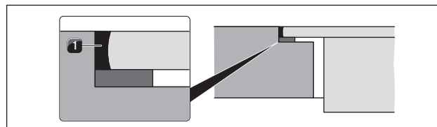
Fig. 5.27 Silicona de sellado para montaje enrasado
