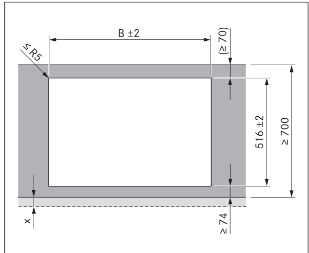
Fig. 5.7 Medidas del recorte para montaje superpuesto
