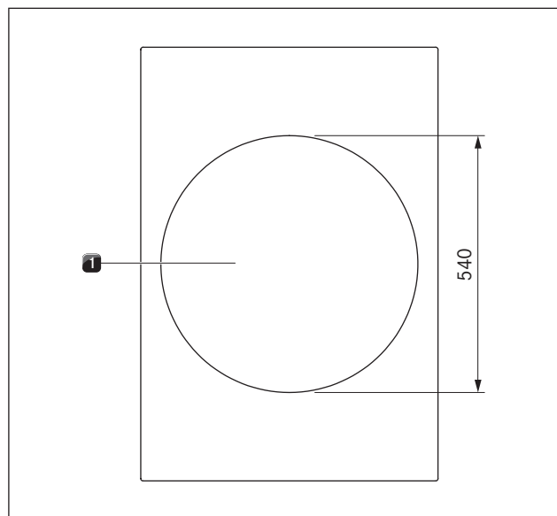
Fig. 4.5 Estructura de la placa PKIW3 y tamaño de la zona de cocción
