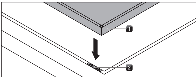
Fig. 5.19 Placa de cocción y placas de compensación de altura
