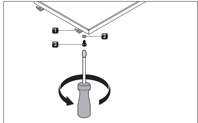
Fig. 5.20 Clips de sujeción
