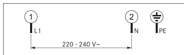
Fig. 5.26 Tilslutningsdiagram 1-faset
