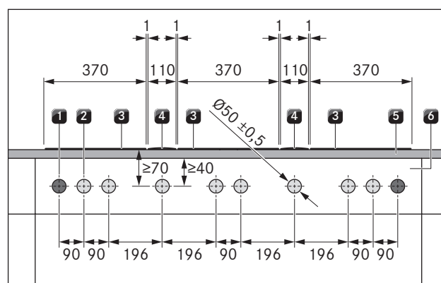
Fig. 5.13 Borebillede, pladeborehuller til 3 kogeplader, 2 emfang og 2 stikdåser
