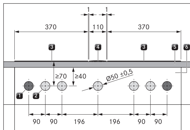
Fig. 5.12 Borebillede, pladeborehuller til 2 kogeplader, 1 emfang og 2 stikdåser
