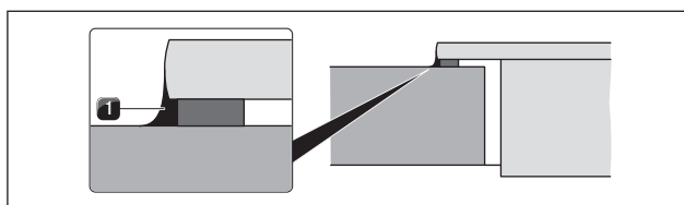
Fig. 5.28 Silikonmasse ved overflademontering
