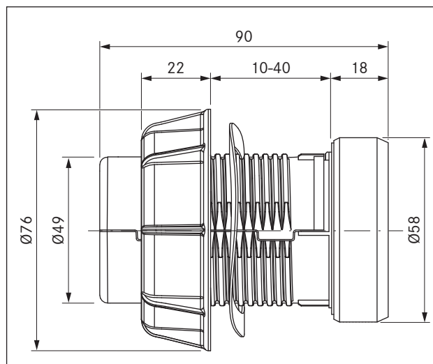
Fig. 3.5 Apparatmål betjeningsknop
