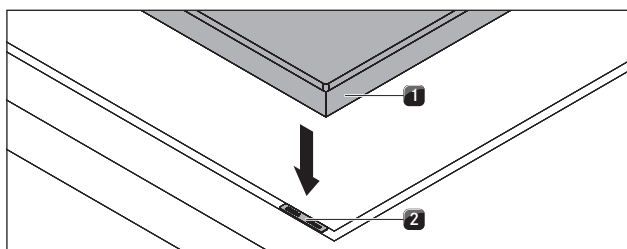
Fig. 5.19 Kogeplade og højdeudligningsplader
