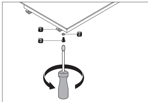
Fig. 5.20 Fastgørelsesclips
