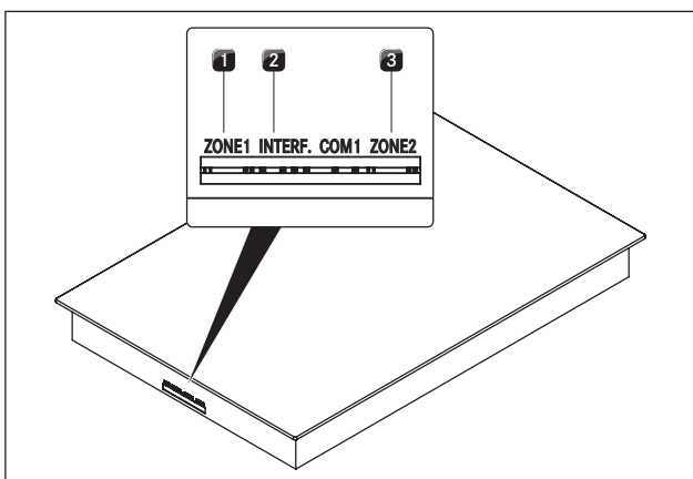
Fig. 5.22 Tilslutninger på kogepladen
