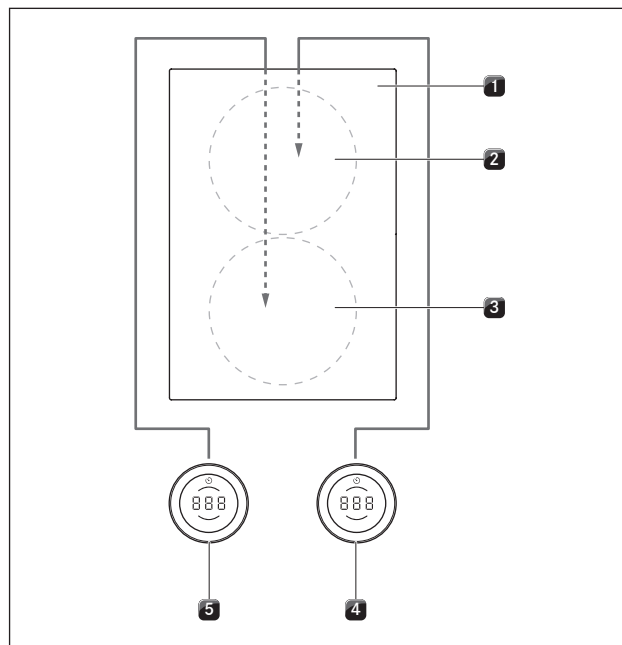
Prikaz 5.22 Priključak zona za kuhanje pri ugradnji okrenutoj za 180° i uređajima s priključkom sprijeda
