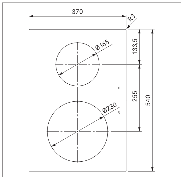
Prikaz 3.1 Dimenzije uređaja PKI3, prikaz odozgo
