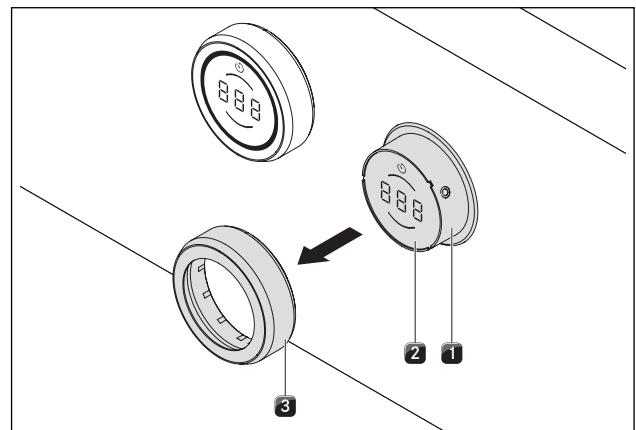
Prikaz 7.1 Skidanje prstena gumba
