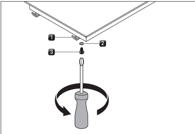
Kuva 5.18 Asennuskannakkeet
