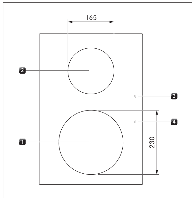
Kuva 4.5 Keittotason PKI3 rakenne ja keittoalueiden koko
