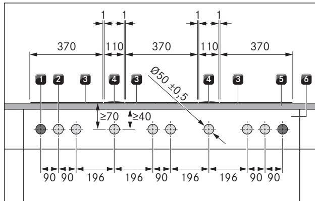
Kuva 5.12 Porauskuva: porausaukot kolmelle keittotasolle, kahdelle keittotason höyrynpöistölle ja kahdelle pistorasialle
