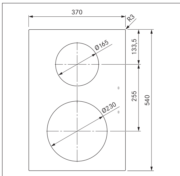
Kuva 3.1 Laitemitat PKI3 kuva ylhäältä
