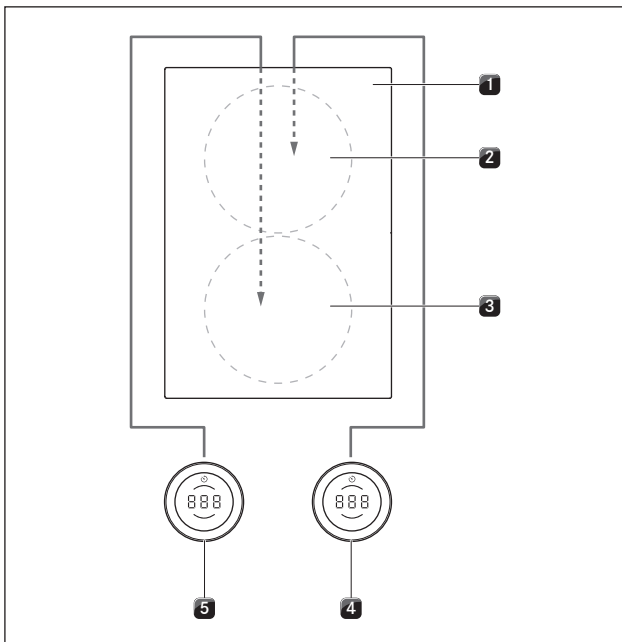
Kuva 5.22 Keittoalueiden liitanta 180° käänteisessä asennuksessa ja laitteissa, joissa liitanta edessä
