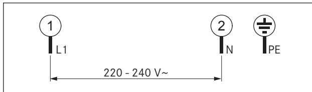
Abb. 5.24 Anschlussschema 1-phasig
