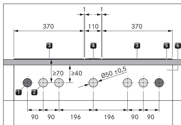
bild 5.15 Borrbild borrhning av lister för 2 spishällar, 1 ångsug och 2 kontaktuttag
