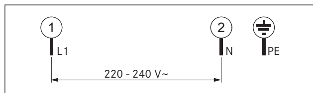
bild 5.33 Kopplingschema 1-fasigt
