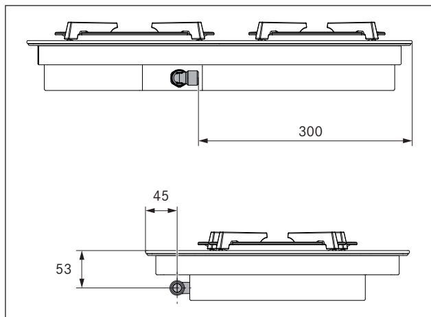
bild 5.20 Position gasanslutning
