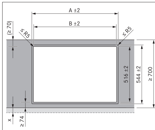
bild 5.9 Ursparningsmått för planmontering
