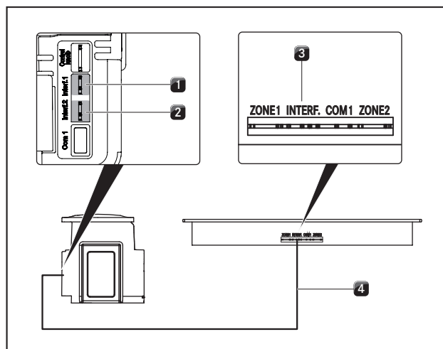
Ilustracja 4.32 Ustawianie komunikacji między wyciągiem oparów i płytami grzewczymi
