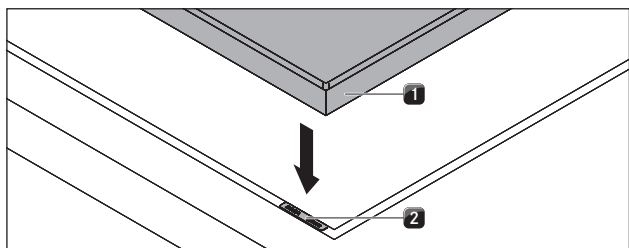
Ilustracja 4.25 Płyta grzewcza i podkładki wyrównujące
