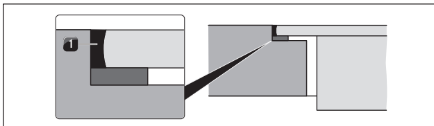
Ilustracja 4.34 Masa silikonowa przy montażu z zachowaniem równej powierzchni
