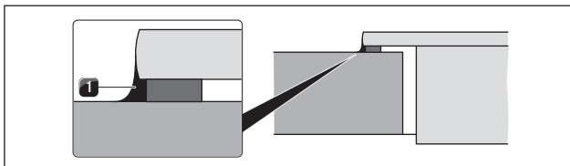
Ilustracja 4.35 Masa silikonowa przy montażu elementu z uskokiem
