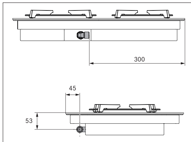
Ilustracja 4.20 Położenie przyłącza gazu
