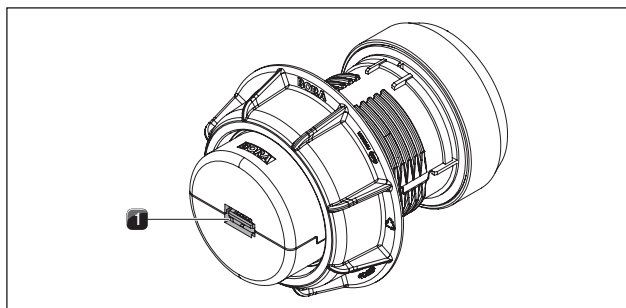
Ilustracja 4.28 Tylne pole grzewcze z przyłączem
