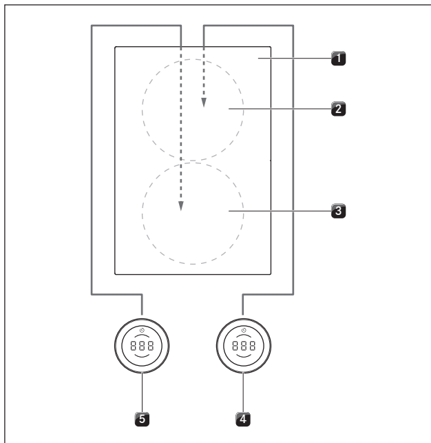
Ilustracja 4.31 Przyłączanie pól grzewczych dla montażu w pozycji obróconej o 180° i urządzeń z przyłączami z przodu
