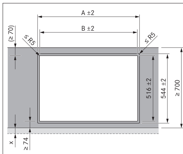
Ilustracja 4.9 Wymiary wycięcia dla montażu z zachowaniem równej powierzchni
