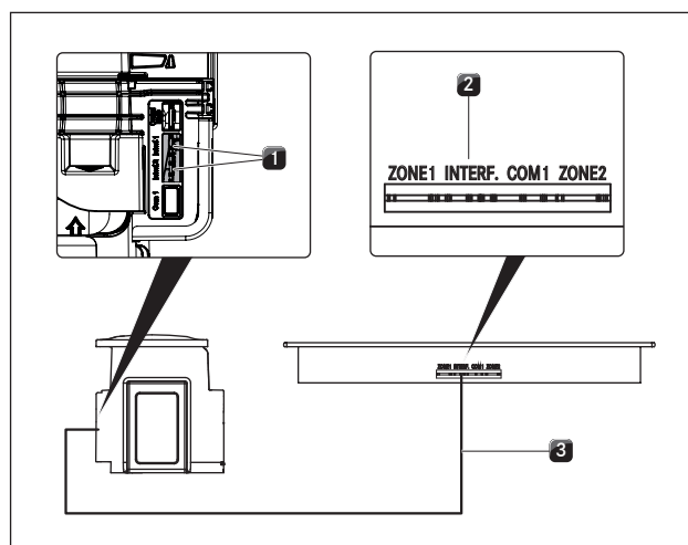
Ilustracja 5.26 Ustawianie komunikacji między wyciągiem oparów i płytami grzewczymi
