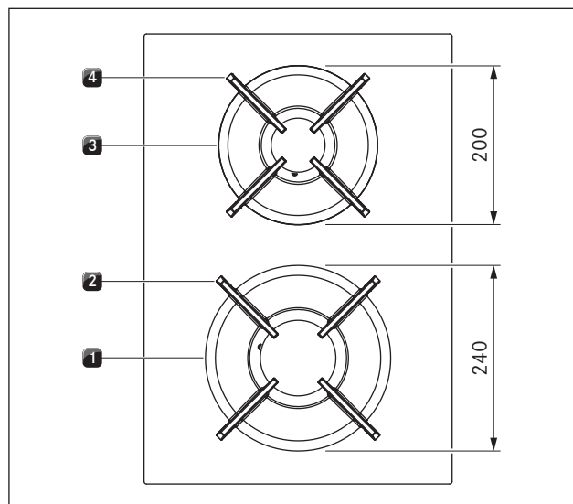
Ilustracja 4.5 Budowa gazowej płyty grzewczej PKG3 i wielkość pól grzewczych
