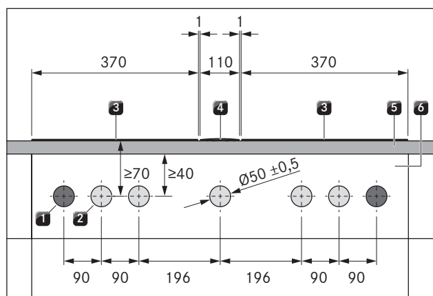
Ilustracja 5.14 Rozmieszczenie otworów w przesłonie dla 2 płyt grzewczych, 1 wyciągu oparów i 2 gniazdek
