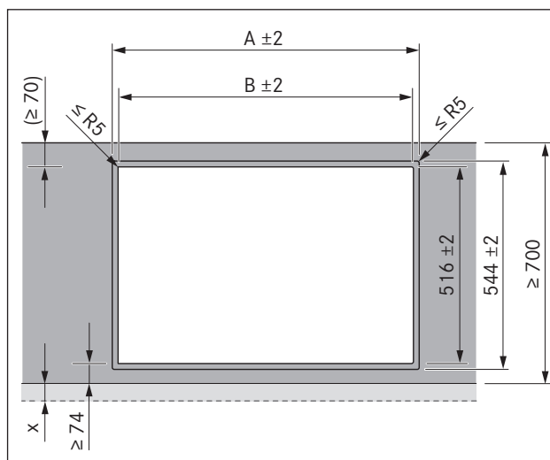
Ilustracja 5.8 Wymiary wycięcia dla montażu z zachowaniem równej powierzchni
