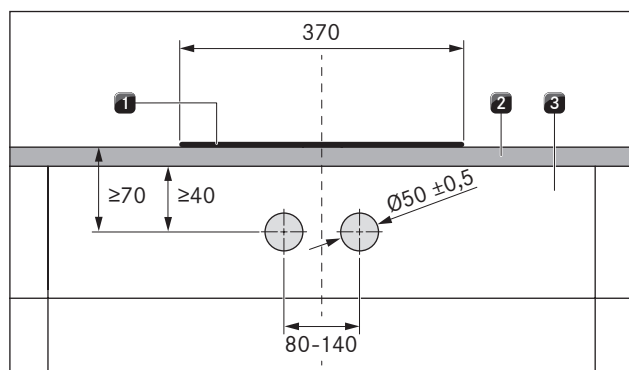
Ilustracja 5.13 Rozmieszczenie otworów w przesłonie płyt grzewczych
