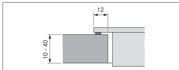
Ilustracja 5.11 Wymiary podparcia dla montażu elementu z uskokiem
