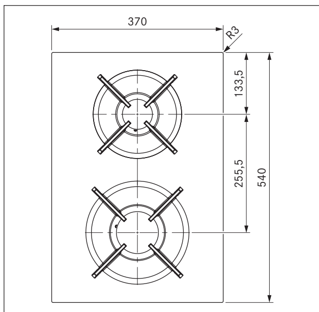
Ilustracja 3.1 Wymiary urządzenia PKG11 – widok z góry
