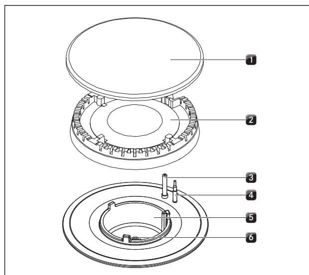
Ilustracja 5.28 Budowa palnika gazowego
