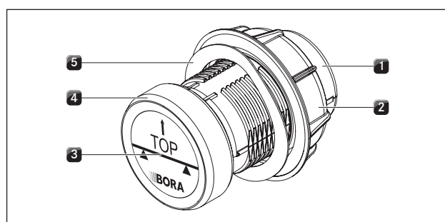
Ilustracja 5.16 Budowa gałki obsługi
