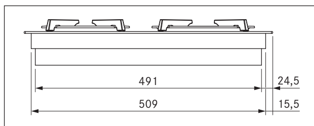
Ilustracja 3.3 Wymiary urządzenia PKG11 – widok z boku
