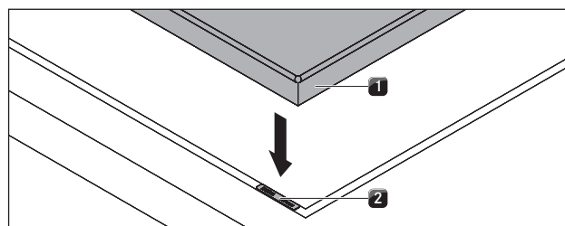
Ilustracja 5.20 Płyta grzewcza i podkładki wyrównujące
