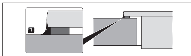
Ilustracja 5.32 Masa silikonowa przy montażu elementu z uskokiem
