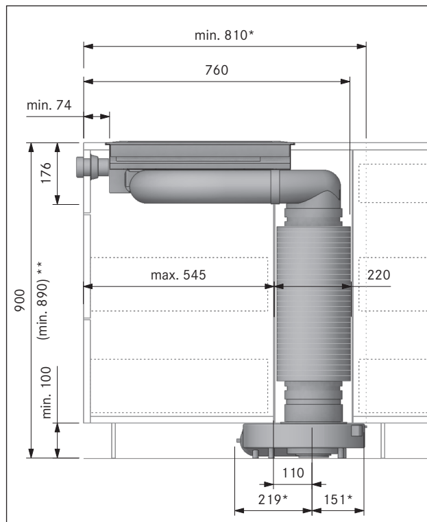
Ilustracja 5.3 Wymiary zabudowy urządzenia PKA3/PKA3AB z okrągłym tłumikiem hałasu USDR50 przy budowie standardowej
