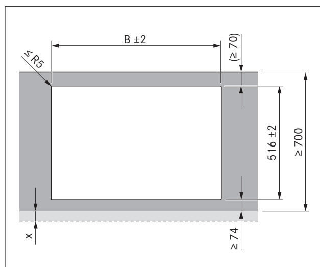
Ilustracja 5.10 Wymiary wycięcia dla montażu elementu z uskokiem
