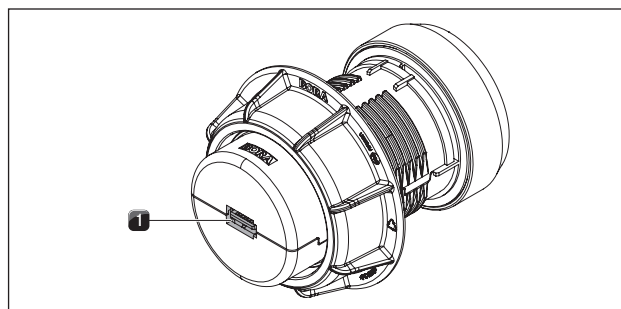
Ilustracja 5.22 Tylna strona gałki obsługi z przyłączem
