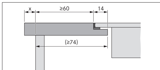
Ilustracja 5.7 Wystający na zewnątrz odcinek blatu
