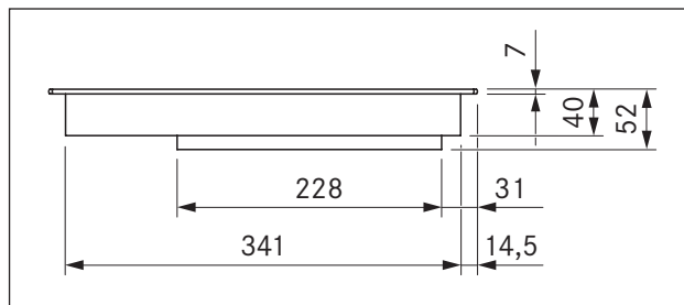
Ilustracja 3.2 Wymiary urządzenia PKG11 – widok z przodu
