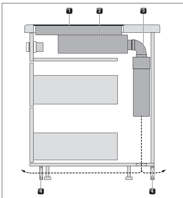
Ilustracja 5.6 Przykład rozplanowania dla odprowadzania powietrza w obiegu zamkniętym (wyspa kuchenna + PKG3 + PKAS3 + jednostka oczyszczająca powietrze)
