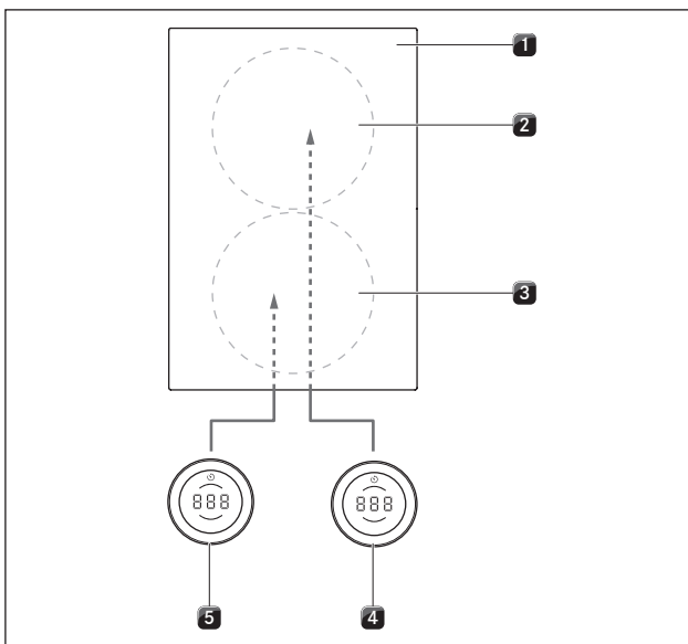
Abb. 5.30 Standaardaansluiting bij apparaten met aansluiting vooraan
