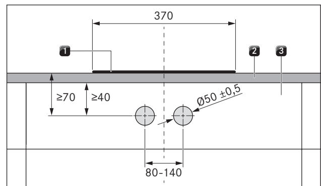
Abb. 5.14 Boorschema voor de boorgaten in het paneel voor de kookvelden
