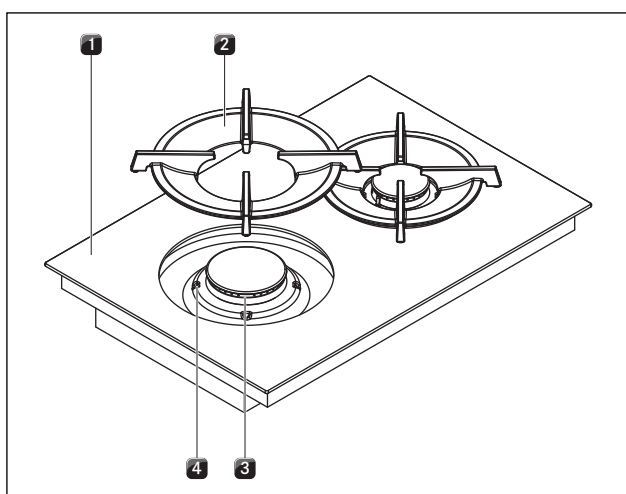
Afb. 8.1 Opbouw gasbrander
