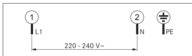
Abb. 5.33 Aansluitschema 1-fasig
