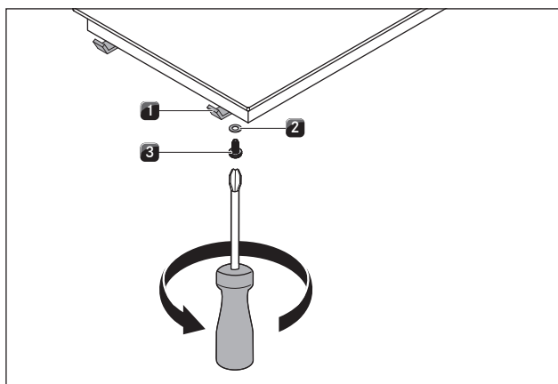
Abb. 5.26 Bevestigingsklemmen
