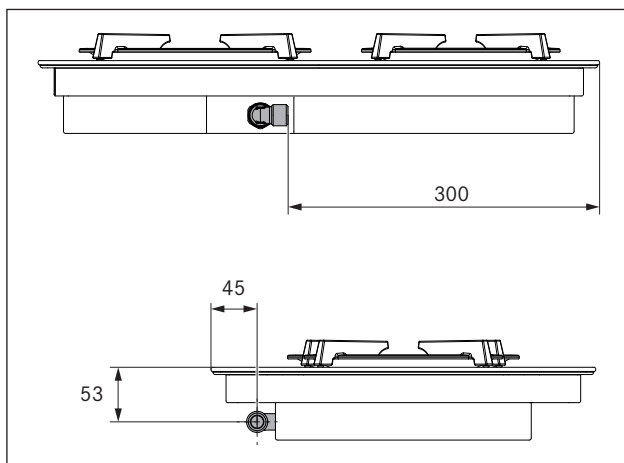
Abb. 5.20 Positie gasaansluiting
