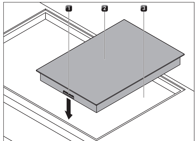
Abb. 5.24 Kookveld plaatsen
