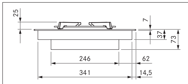
Afb. 3.2 PKG3 toestelafmetingen vooraanzicht
