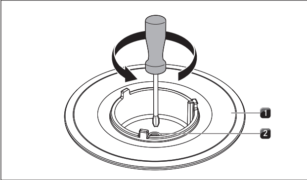
Abb. 5.22 Kookplaatbrander met gassproeier
