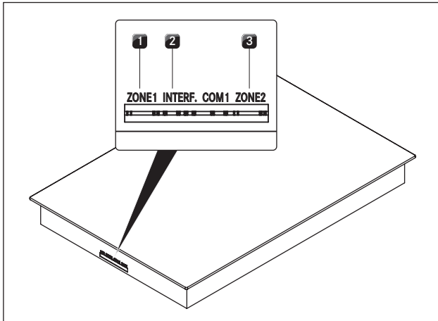
Abb. 5.29 Aansluitingen op het kookveld
