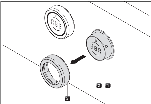
Afb. 8.3 Knopring verwijderen
