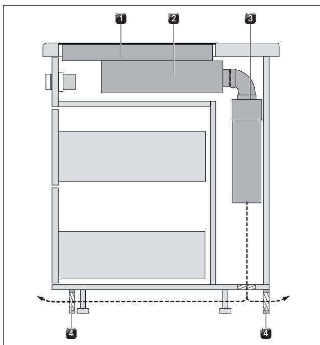
Abb. 5.7 Ontwerpvoorbeeld bij systeem met luchtrecirculatie (keukeneiland + PKG3 + PKAS3 + luchtreinigingseenheid)
