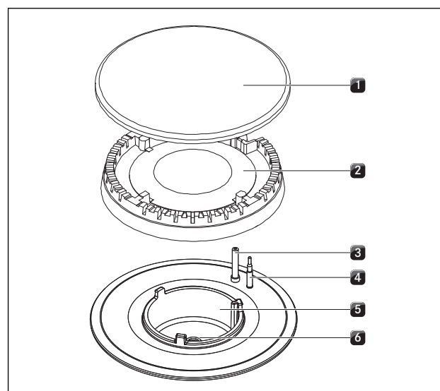
Abb. 5.21 Opbouw gasbrander
