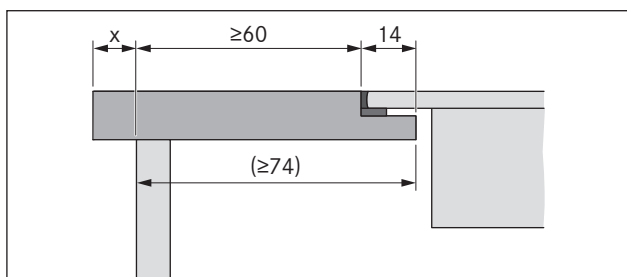
Abb. 5.8 Uitstekend deel van het werkblad
