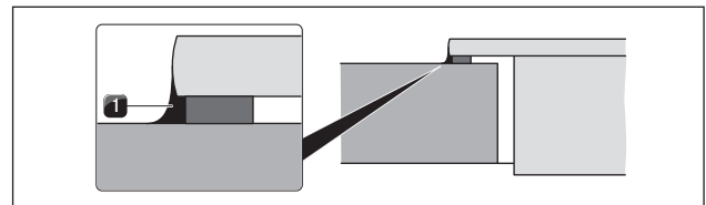
Abb. 5.35 Siliconenkit bij opbouwmontage
