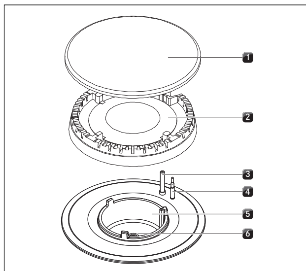
Afb. 8.2 Opbouw gasbrander
