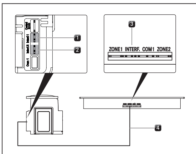
Abb. 5.32 Communicatie tot stand brengen tussen kookveldafzuiging en kookvelden
