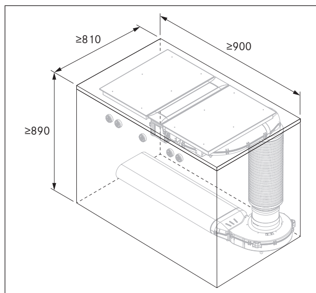
Abb. 5.2 Minimale inbouwafmetingen PKA3/PKA3AB bij standaardopbouw
