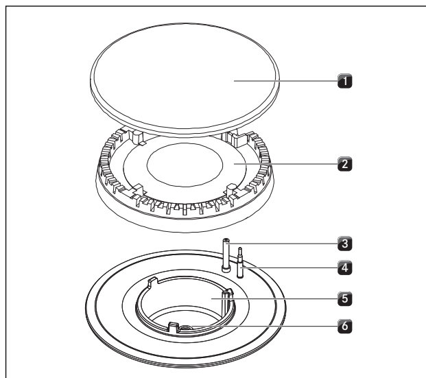
Abb. 5.21 Dijelovi plinskog plamenika
