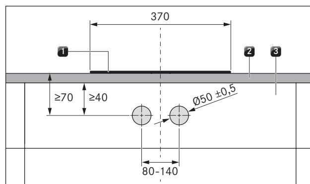
Abb. 5.14 Slika bušenja provrta otvora za ploče za kuhanje
