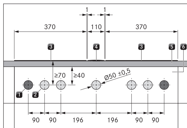
Abb. 5.15 Slika bušenja provrta otvora za 2 ploče za kuhanje, 1 odvod pare i 2 utičnice
