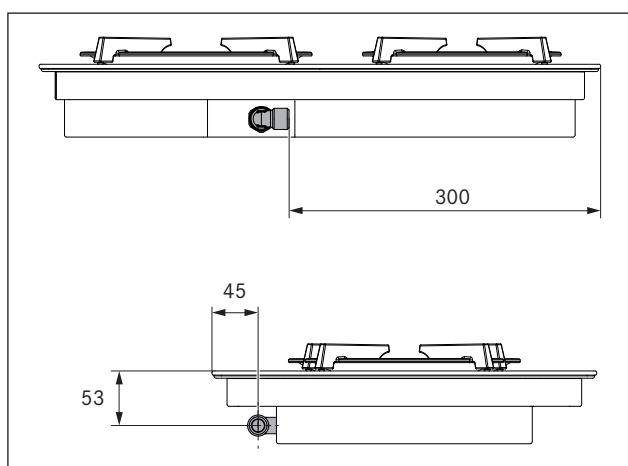
Abb. 5.20 Položaj plinskog priključka
