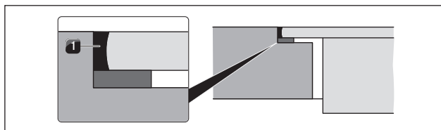
Abb. 5.34 Silikonska masa za brtvljenje pri montaži u ravnini s površinom
