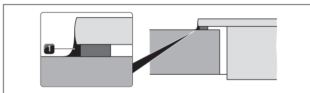
Abb. 5.35 Silikonska masa za brtvljenje pri montaži na površinu
