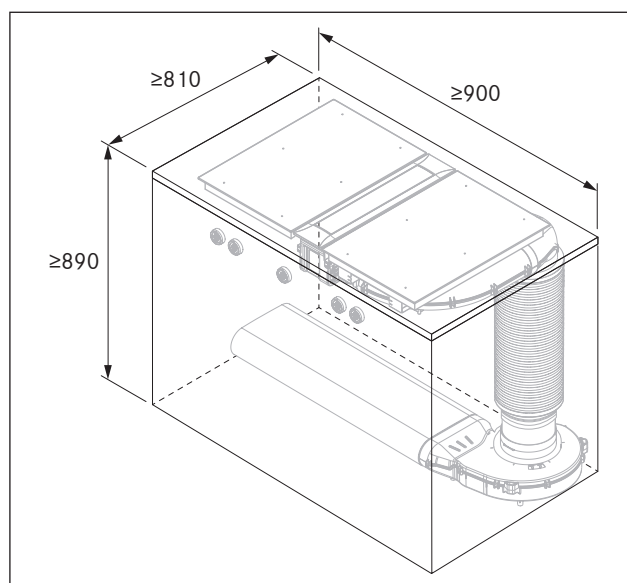
Abb. 5.2 Najmanje dimenzije za ugradnju PKA3/PKA3AB pri standardnoj izvedbi
