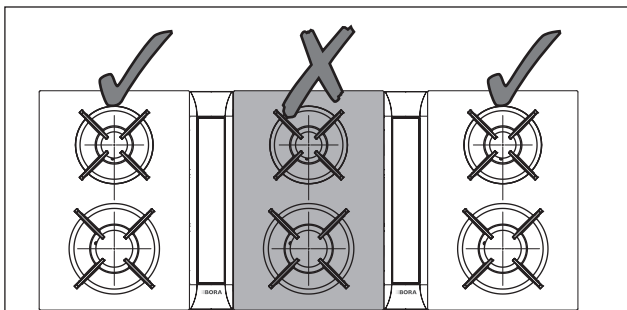
Abb. 5.4 Pozicioniranje plinske ploče za kuhanje PKG3 s dva odvoda pare
