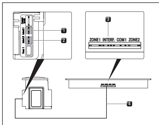
Abb. 5.32 Uspostava komunikacije između odvoda pare i ploča za kuhanje
