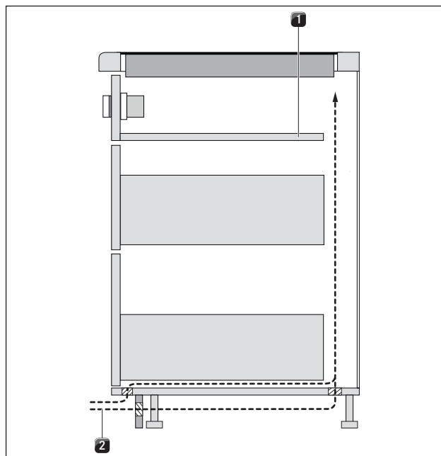
Kuva 5.6 Ilmansyöttö sokkelialue
