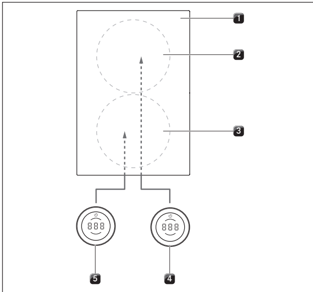
Kuva 5.30 Vakioliitäntä laitteissa, joissa liitäntä edessä
