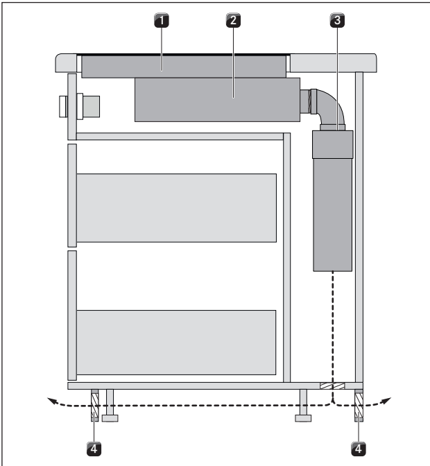
Kuva 5.7 Suunniteluesimerkki kiertoilman takaisin johtamista varten (keittiösaareke + PKG3 + PKAS3 + ilmanpuhdistusyksikkö)
