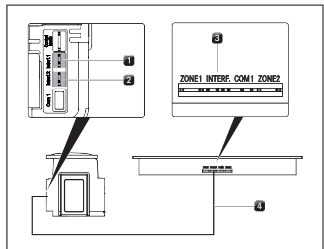
Kuva 5.32 Keittotason höyrynpoiston ja keittotasojen välisen tiedonsiirron muodostaminen
