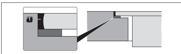
Kuva 5.34 Silikonitiivistysmassa uppoasennuksessa
