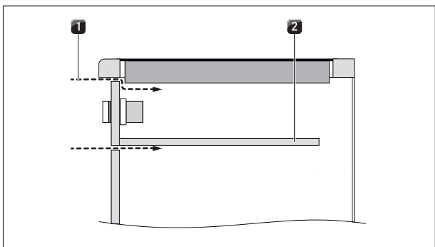
Kuva 5.5 Ilmansyöttö kaappitilan etuosasta
