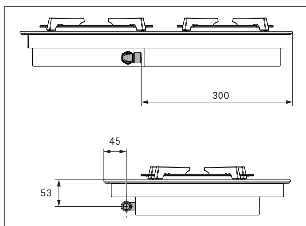
Kuva 5.20 Kaasuliitäntä-asento
