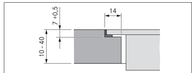
Kuva 5.10 Saumamitta uppoasennusta varten
