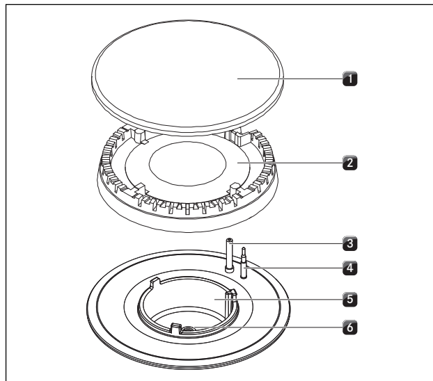
Kuva 8.2 Kaasupolttimen rakenne
