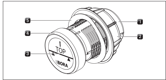
Fig. 5.17 Estructura del mando selector
