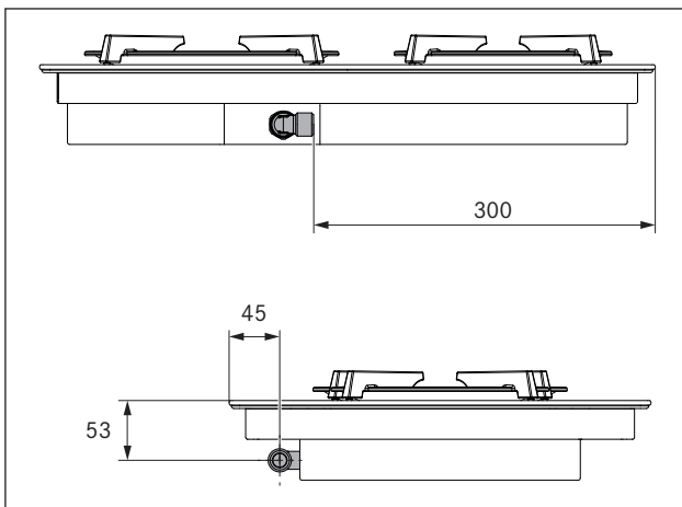
Fig. 5.20 Posición de la toma de gas
