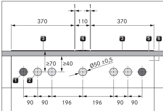
Fig. 5.15 Diagrama de orificios del panel para 2 placas de cocción, 1 extractor de superficie y 2 cajas de enchufe
