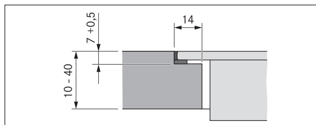
Fig. 5.10 Medida del rebaje para un montaje enrasado
