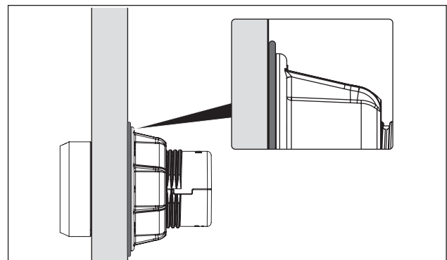
Fig. 5.19 Anillo elástico tras el montaje
