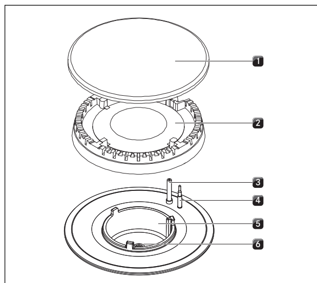
Fig. 5.21 Estructura del quemador de gas
