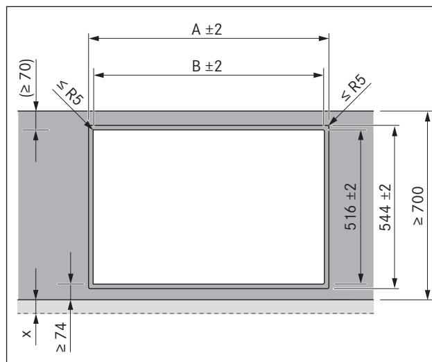
Fig. 5.9 Medidas del recorte para montaje enrasado
