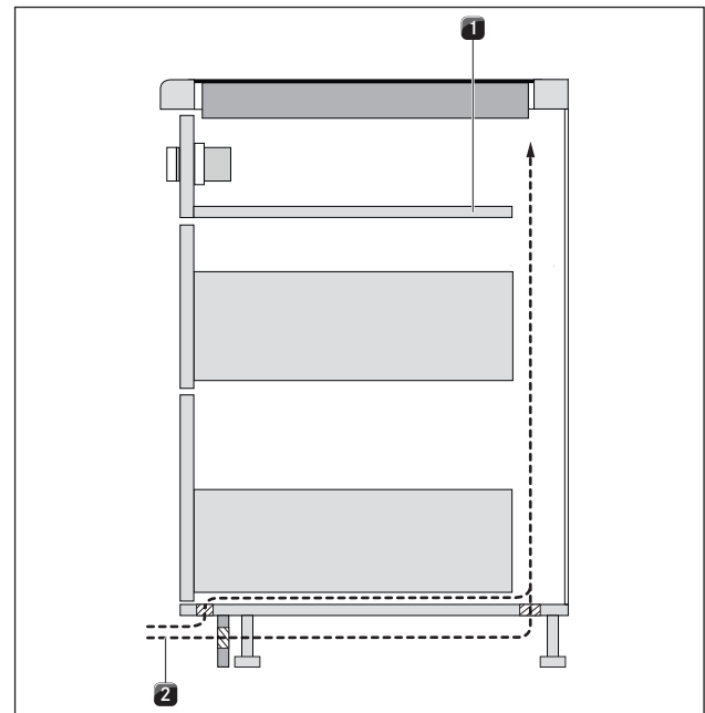
Fig. 5.6 Aporte de aire a la zona del zócalo
