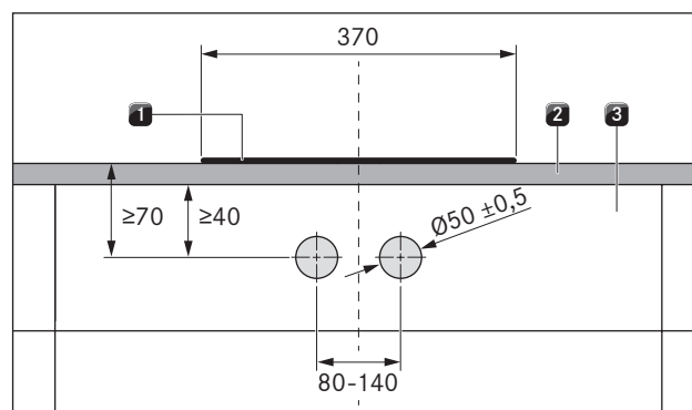
Fig. 5.14 Diagrama de los orificios del panel, placas de cocción
