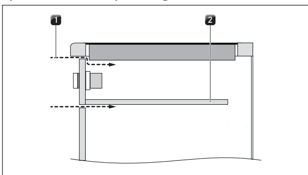
Fig. 5.5 Aporte de aire frontal del módulo
