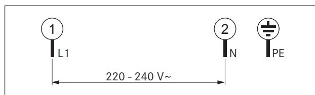
Fig. 5.33 Esquema de conexión monofásica
