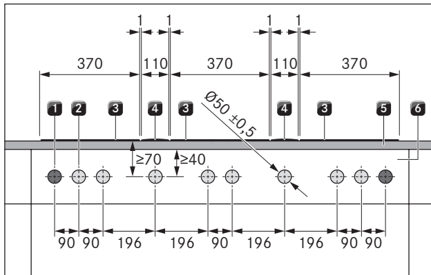
Fig. 5.16 Diagrama de orificios del panel para 3 placas de cocción, 2 extractores de superficie y 2 cajas de enchufe
