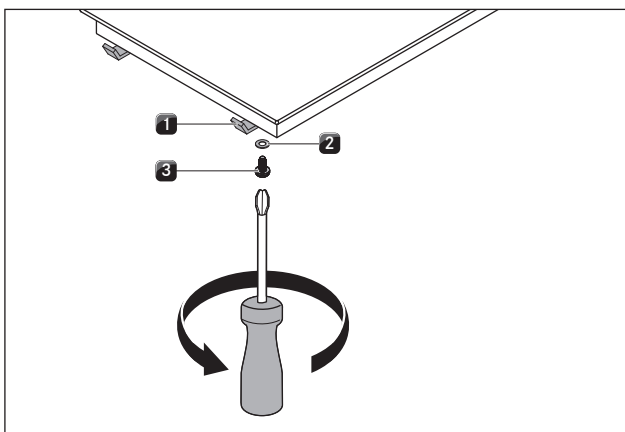
Fig. 5.26 Clips de sujeción
