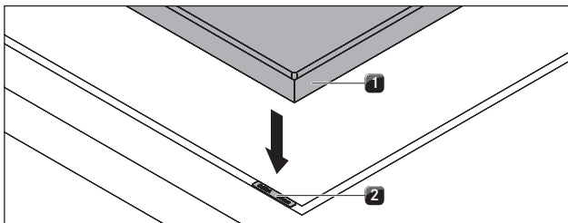
Fig. 5.25 Placa de cocción y placas de compensación de altura
