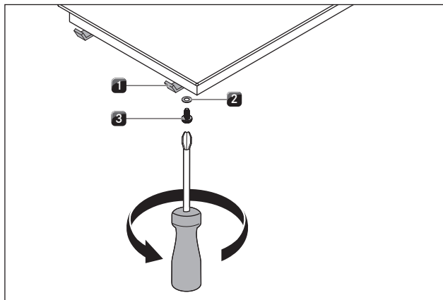
Fig. 5.18 Festeklemmer
