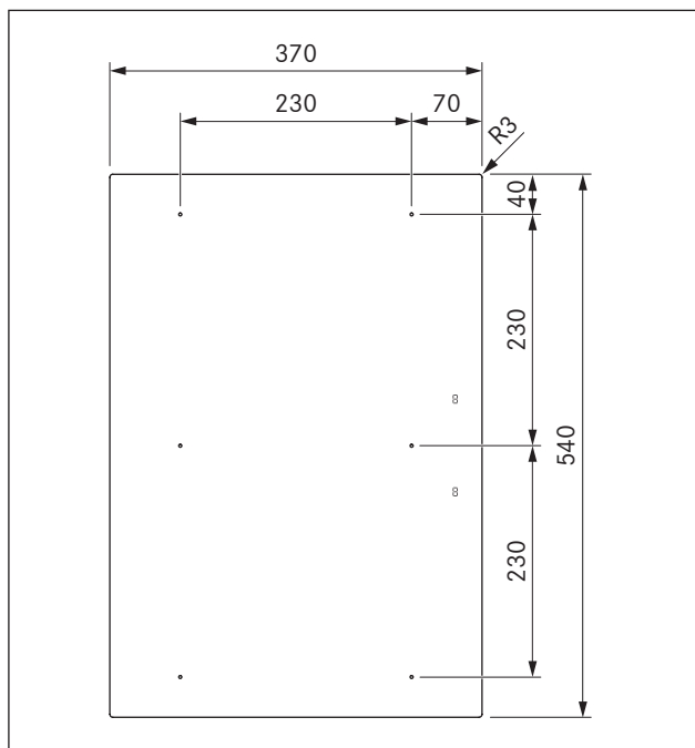
Fig. 3.1 PKFI3 apparatmål visning ovenfra
