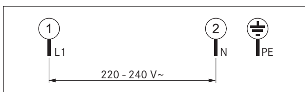
Fig. 5.24 Koble skjema 1-fase
