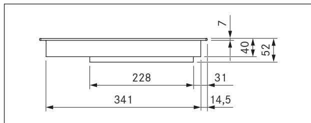
Fig. 3.2 PKFI3 apparatmål visning forfra
