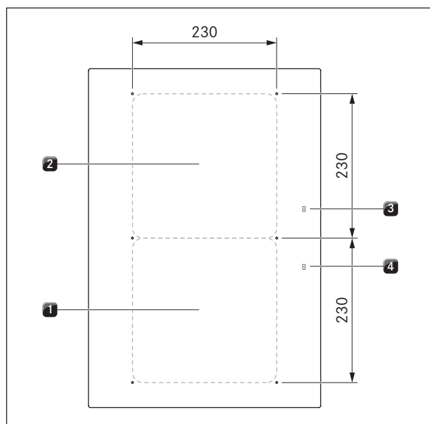
Fig. 4.5 Konstruksjon platetopp PKFI3 og kokesonenes størrelse
