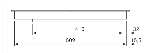
Fig. 3.3 PKFI3 apparatmål visning fra siden
