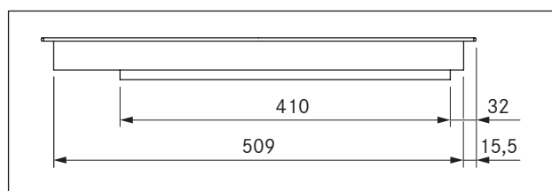
bild 3.3 PKFI3 apparatmått bild från sidan
