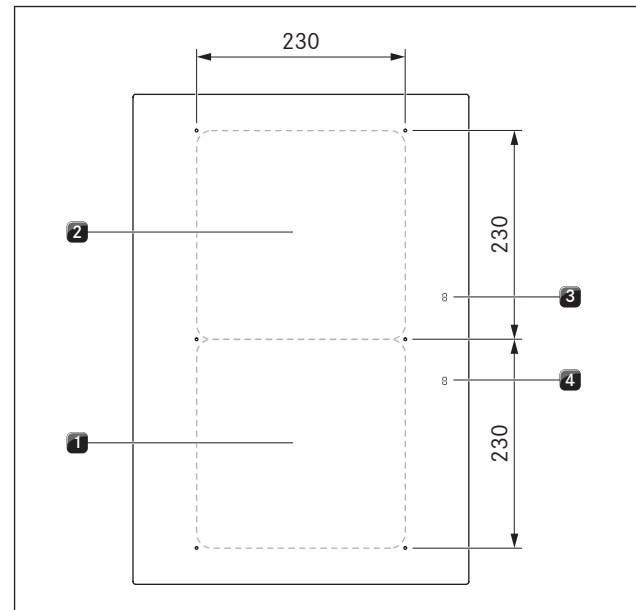
bild 4.5 Konstruktion spishäll PKF13 och storleken på kokzonerna
