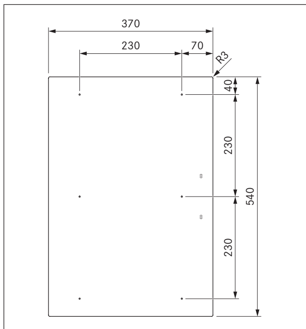
bild 3.1 PKFI3 apparatmått bild från ovan
