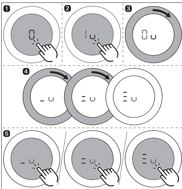
Prikaz 6.10 Aktiviranje funkcije zadržavanja topline (PKFI3, PKI3, PKIW3)
