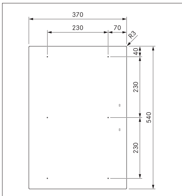
Prikaz 3.1 Dimenzije uređaja PKFI3, prikaz odozgo
