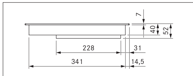
Prikaz 3.2 Dimenzije uređaja PKFI3, prikaz srijeda
