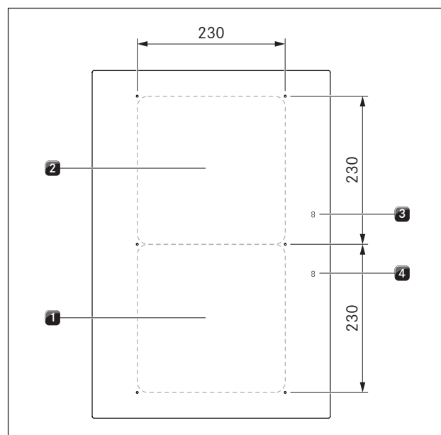
Prikaz 4.5 Dijelovi ploče za kuhanje PKFI3 i veličina zona za kuhanje
