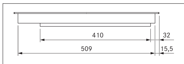
Prikaz 3.3 Dimenzije uređaja PKFI3, bočni prikaz
