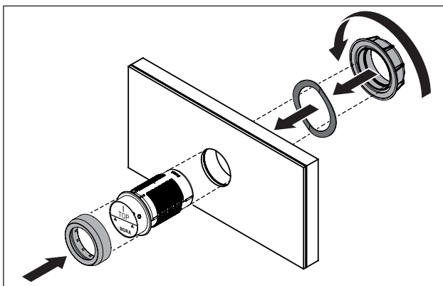
Fig. 4.14 Montage du bouton de commande
