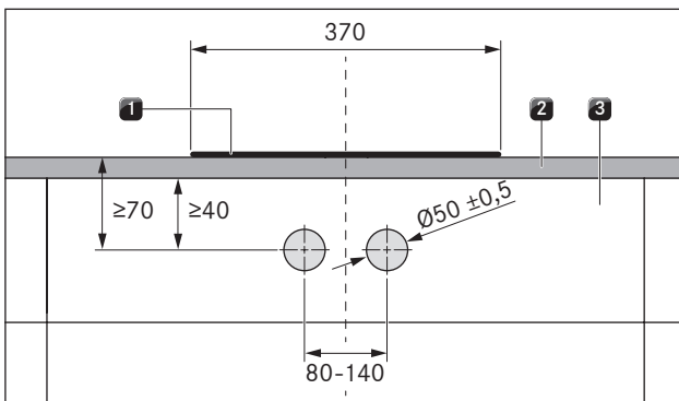
Fig. 4.10 Schéma de perçage du bandeau pour les tables de cuisson
