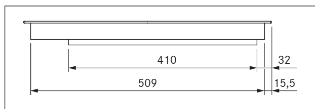
Fig. 3.3 Dimensions PKFI3 - Vue latérale
