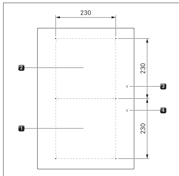
Fig. 5.5 Composition de la table de cuisson PKFI3 et dimensions des zones de cuisson
