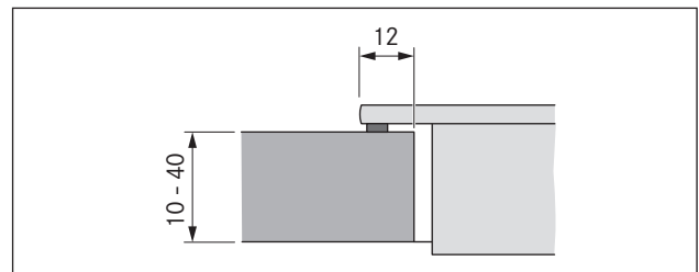
Fig. 4.8 Cote d'appui pour montage en saillie
