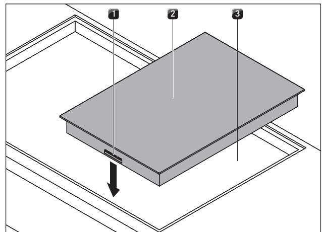
Fig. 4.16 Pose de la table de cuisson
