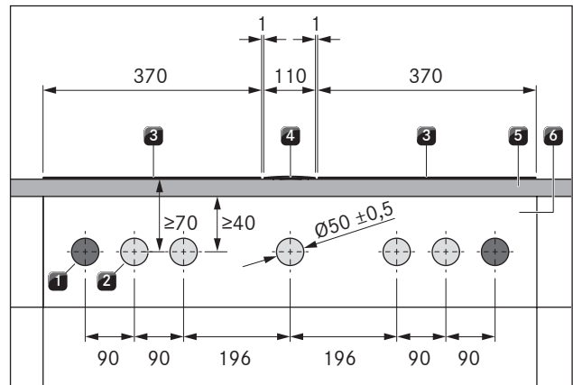
Fig. 4.11 Schéma de perçage du bandeau pour 2 tables de cuisson, 1 dispositif aspirant et 2 prises
