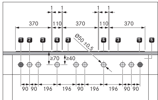
Fig. 4.12 Schéma de perçage du bandeau pour 3 tables de cuisson, 2 dispositifs aspirants et 2 prises
