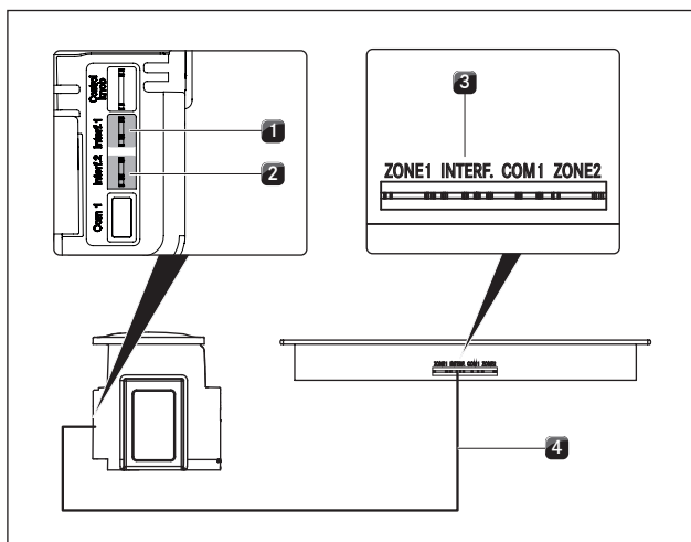
Fig. 4.23 Raccordement de communication entre le dispositif aspirant et les tables de cuisson
