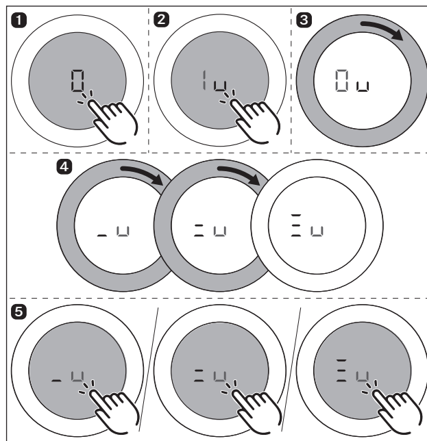
Fig. 6.10 Activation de la fonction de maintien au chaud
