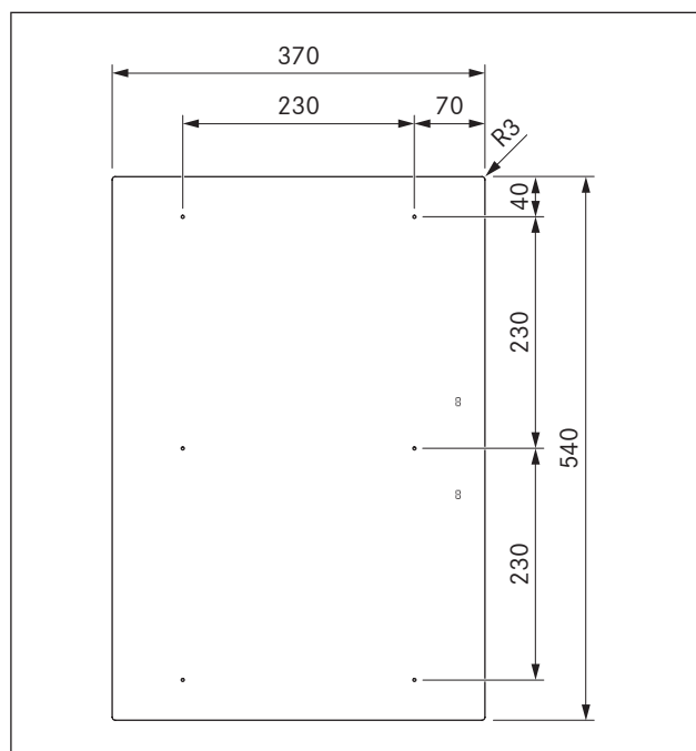
Fig. 3.1 Dimensions PKFI3 - Vue de dessus
