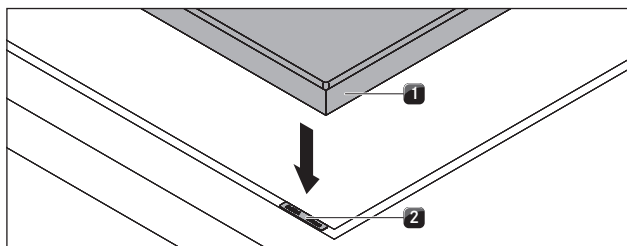
Fig. 4.17 Table de cuisson et plaques de compensation des hauteurs
