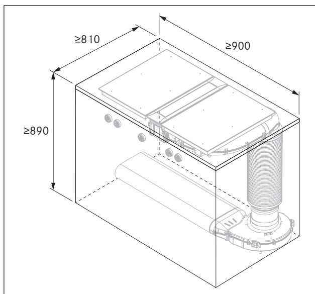
Fig. 4.2 Dimensions minimales de montage pour PKA3/PKA3AB en montage standard
