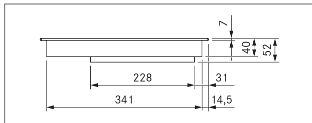
Fig. 3.2 Dimensions PKFI3 - Vue de devant
