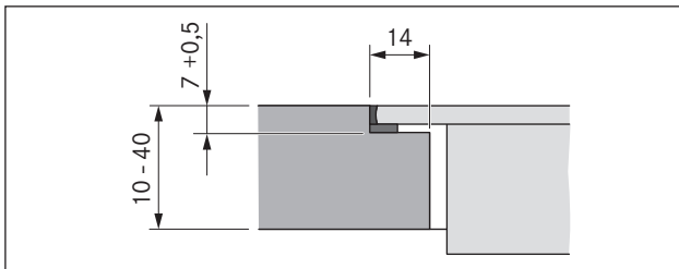
Fig. 4.6 Dimension de rainure pour montage affleurant
