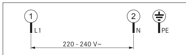
Fig. 4.24 Schéma de raccordement 1 phases
