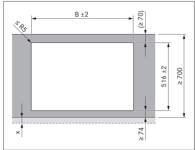
Fig. 4.7 Dimensions de découpe pour montage en saillie
