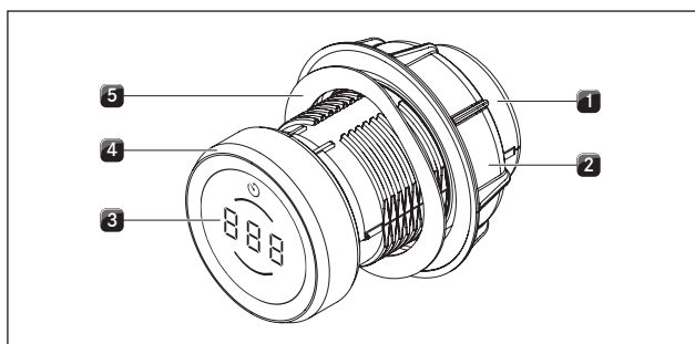
Fig. 5.1 Composition du bouton de commande
