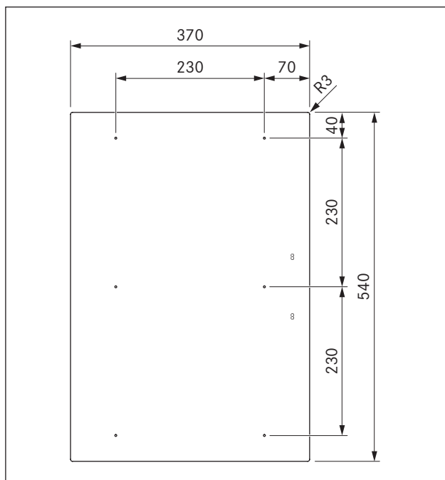
Obr. 3.1 Rozměry produktu PKFI3 – pohled shora
