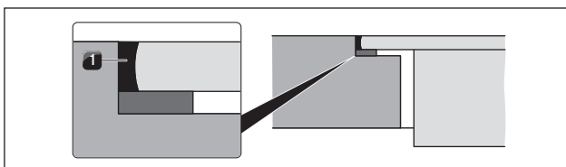
Obr. 5.25 Silikonová těsnicí hmota při plošně zarovnané montáži
