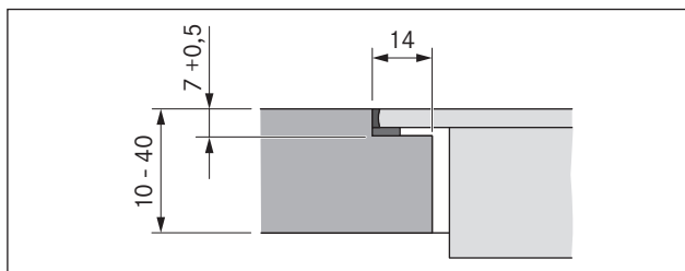
Obr. 5.6 Rozměr drážky pro plošně zarovnanou montáž
