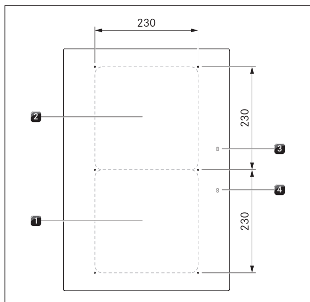
Obr. 4.5 Konstrukce varné desky PKFI3 a rozměry varných zón
