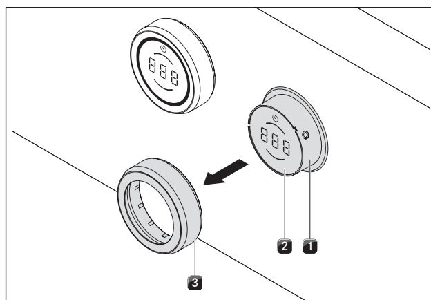
Kuva 7.1 Säätörengaan irtivetäminen
