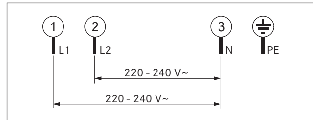
Kuva 5.26 Liitäntäkaavio – 2-vaiheinen liitäntä
