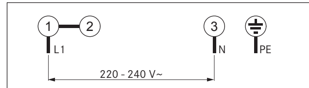
Kuva 5.25 Liitäntäkaavio – 1-vaiheinen liitäntä
