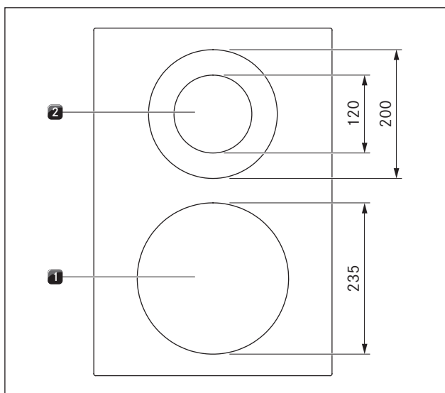
Kuva 4.5 Keittotason PKCH3 rakenne ja keittoalueiden koko
