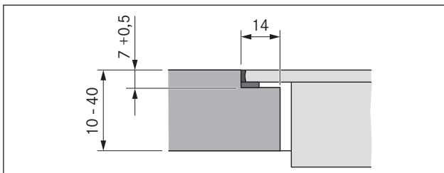
Kuva 5.6 Saumamitta uppoasennusta varten
