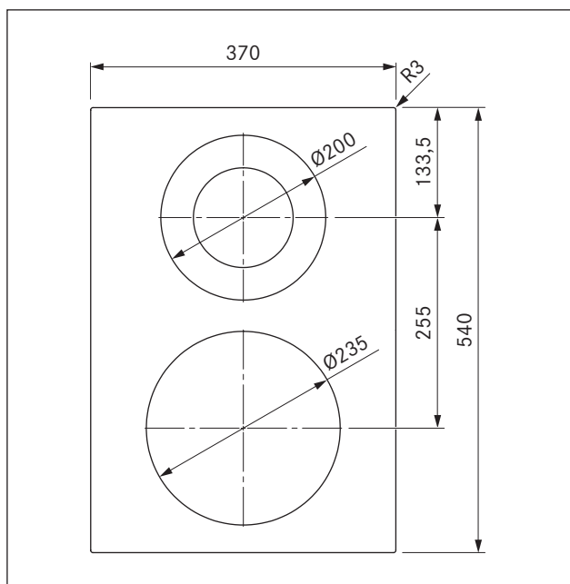
Kuva 3.1 Laitemitat PKCH3 kuva ylhäältä
