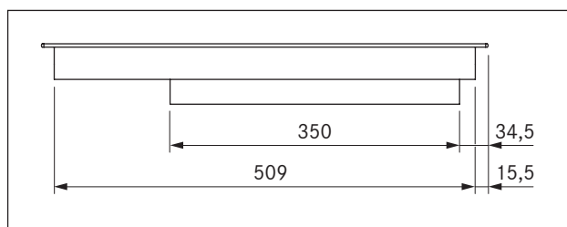
Kuva 3.3 Laitemitat PKCH3 sivukuva
