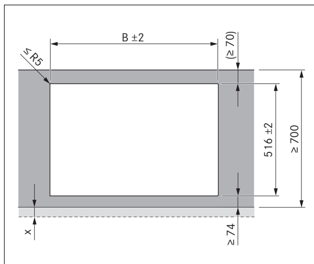
Kuva 5.7 Asennusaukkojen mitat pinta-asennusta varten
