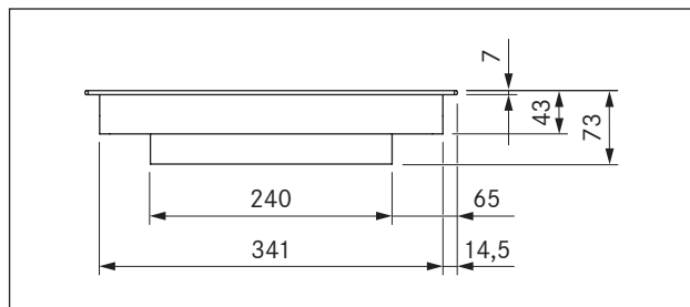
Kuva 3.2 Laitemitat PKCH3 kuva edestä
