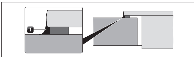
Kuva 5.28 Silikonitiivistysmassa pinta-asennuksessa
