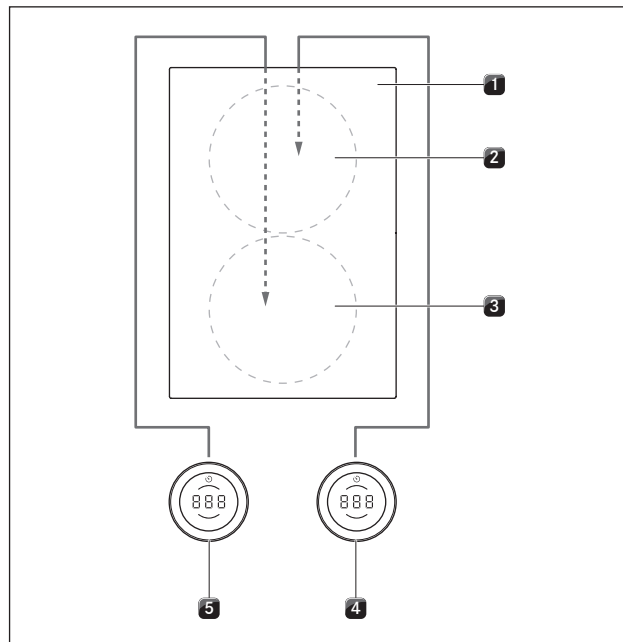
Kuva 5.23 Keittoalueiden liittäntä 180° käänteisessä asennuksessa ja laitteissa, joissa liittäntä edessä
