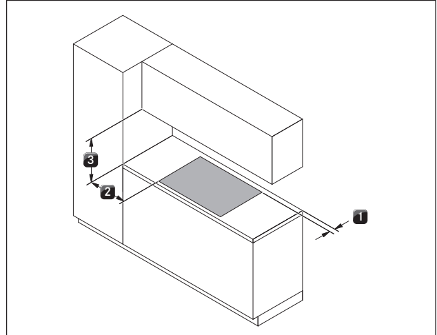
Kuva 5.19 Minimietäisyydet 180° käänteisen asennuksen yhteydessä
